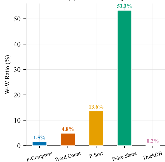
(d) W-W Severity
