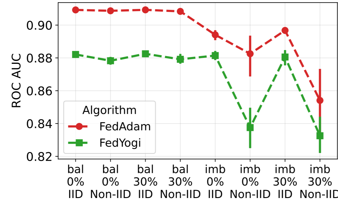
ROC AUC
