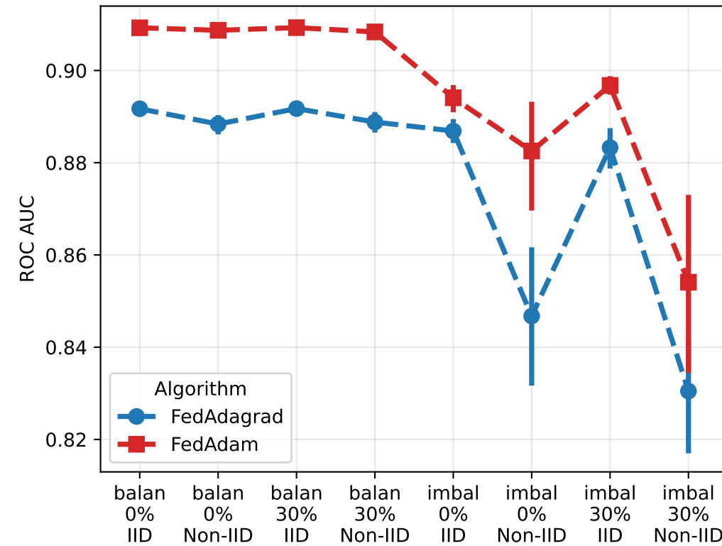
ROC AUC
