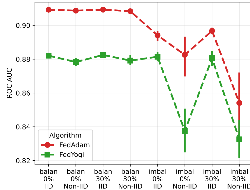
ROC AUC
