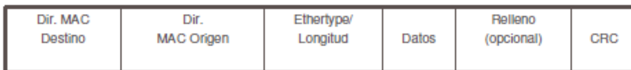
Trama 802.3
