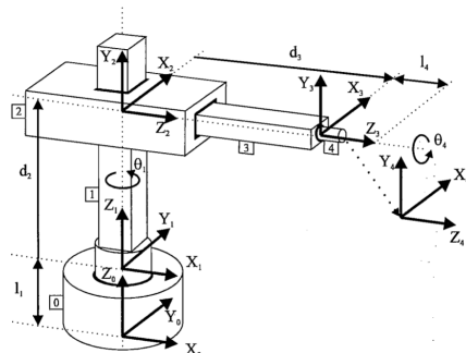
Robot Cilíndrico
