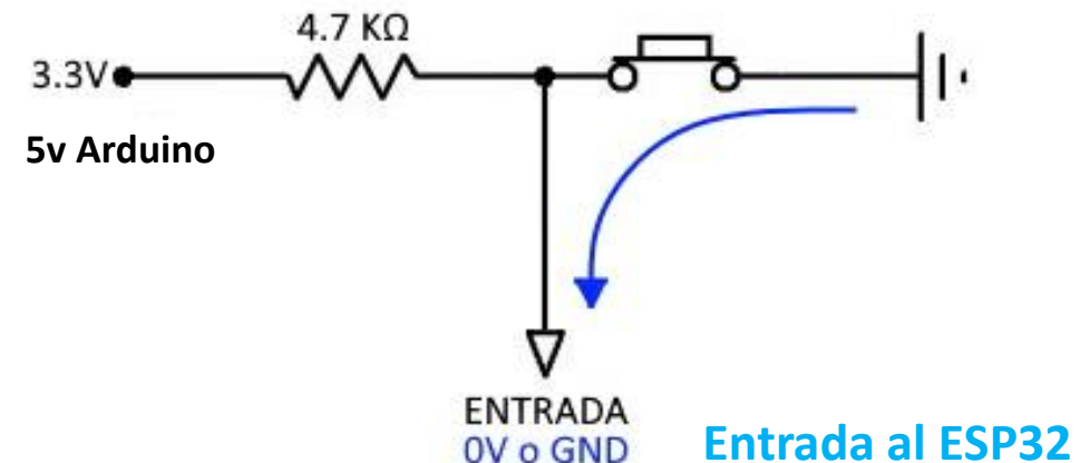
Pulsador cerrado:
