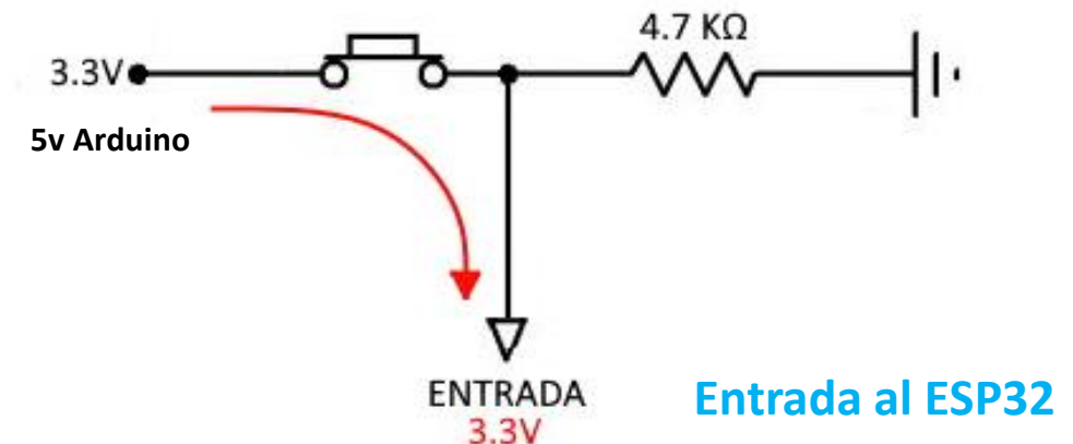
Pulsador cerrado:
