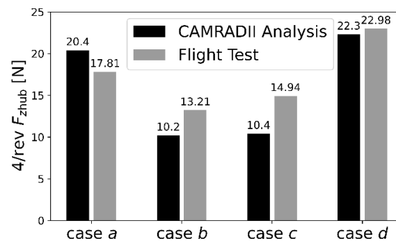
Fig.3.1: CAMRAD II と飛行試験の F_{z\text{hub}} の比較
