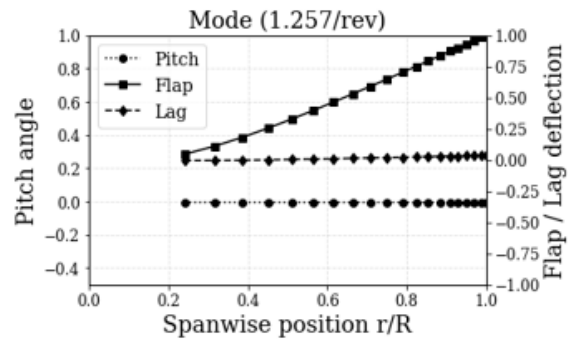
(ii) フラップ 1 次
