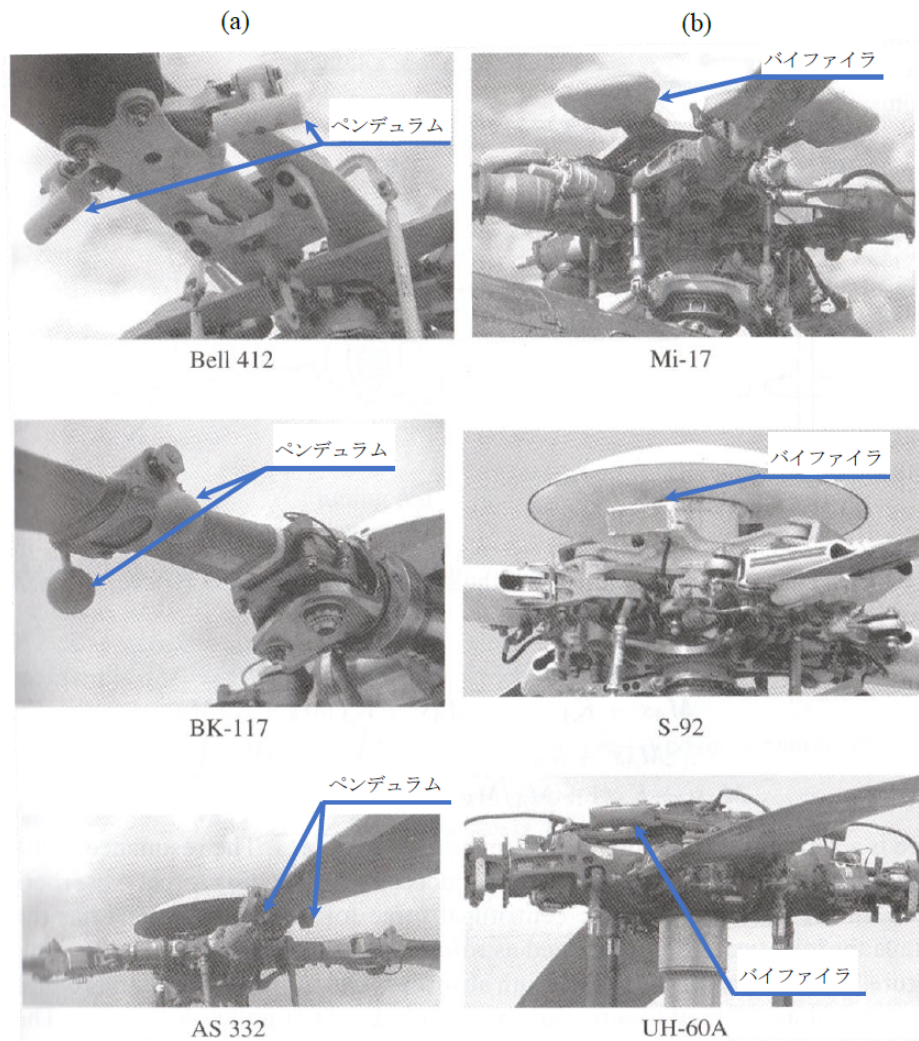
Fig.1.8: ペンデュラムおよびバイファイラ [12]
