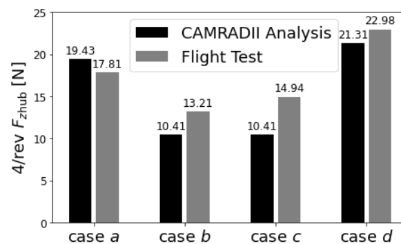
Fig.3.1: CAMRAD II と飛行試験の F_{z\text{hub}} の比較
