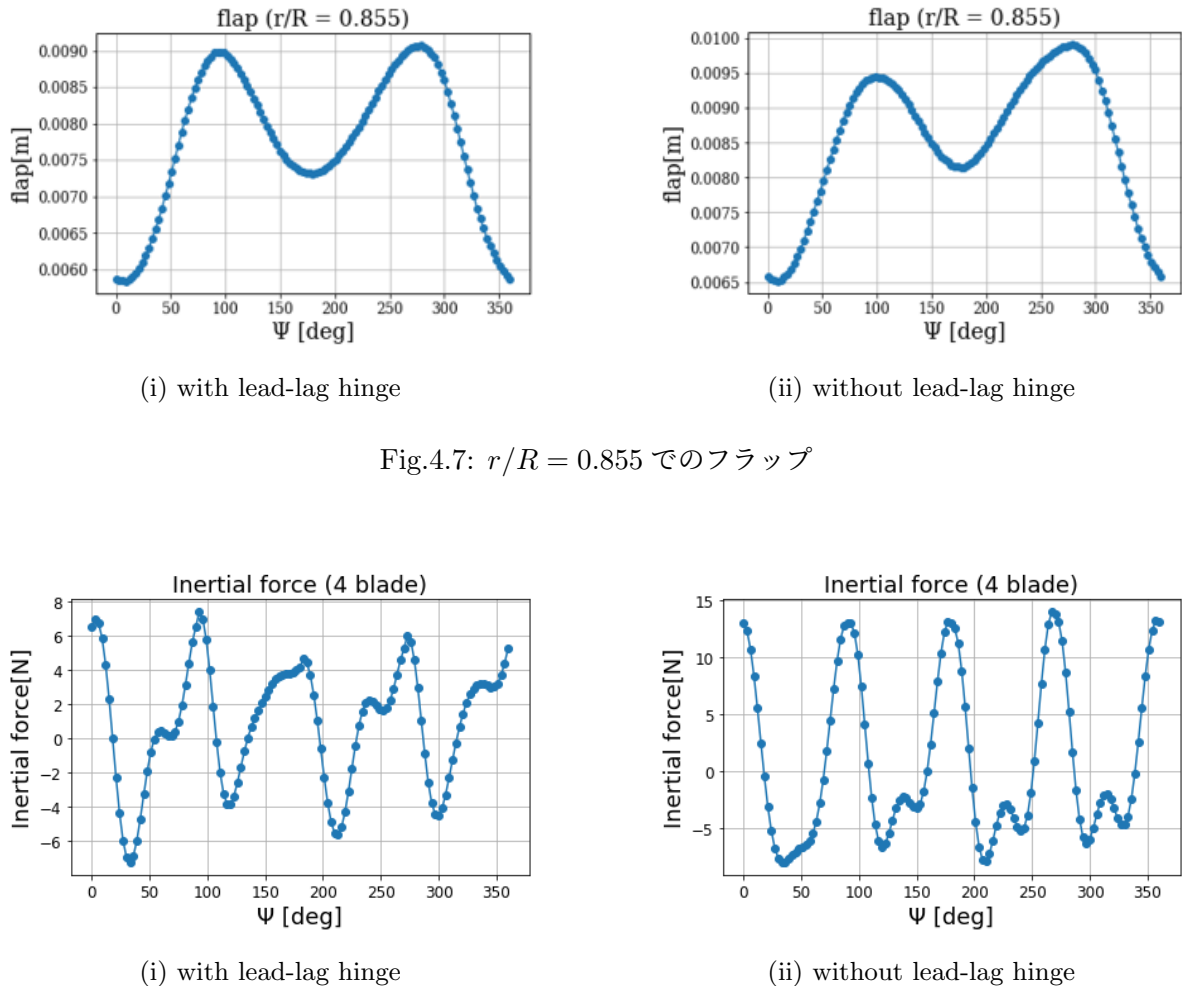
Fig.4.8: 方位角 \Psi と慣性力の関係 (4 ブレード)
