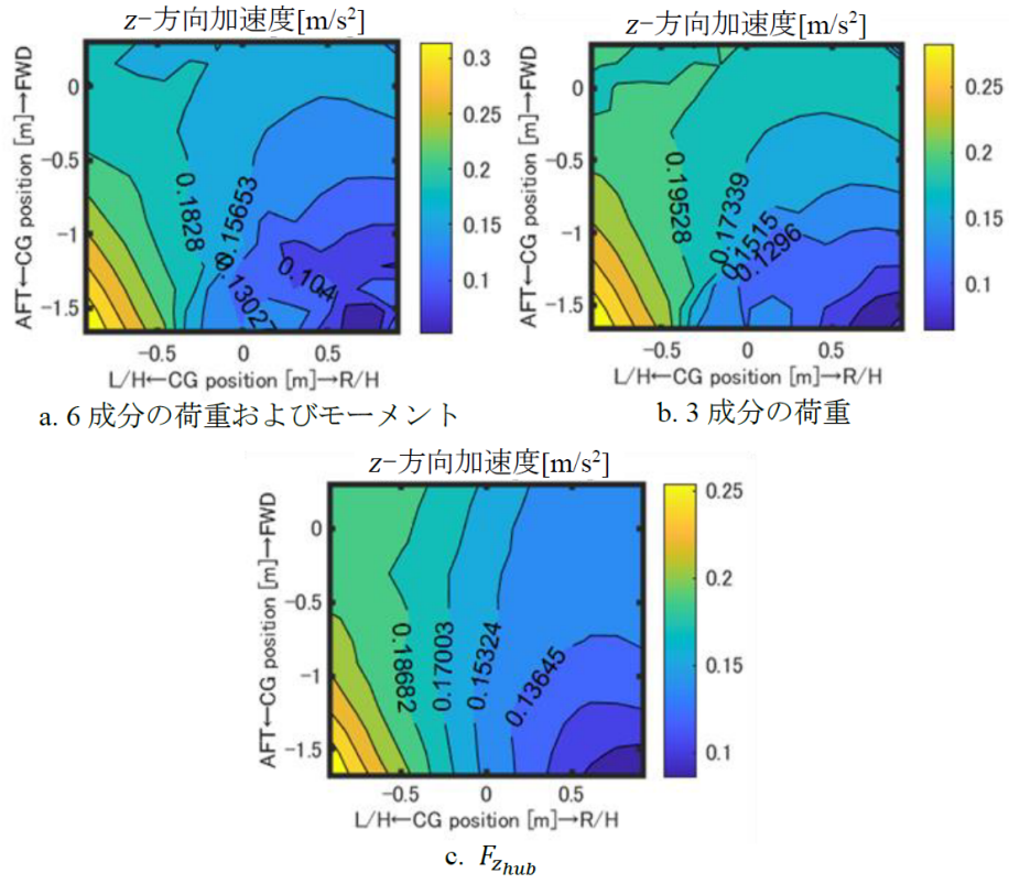
Fig.A.9: パイロット座席での 4/rev z 方向加速度の比較 ( V_c = 61.7 \text{ m/s} ) [15]
