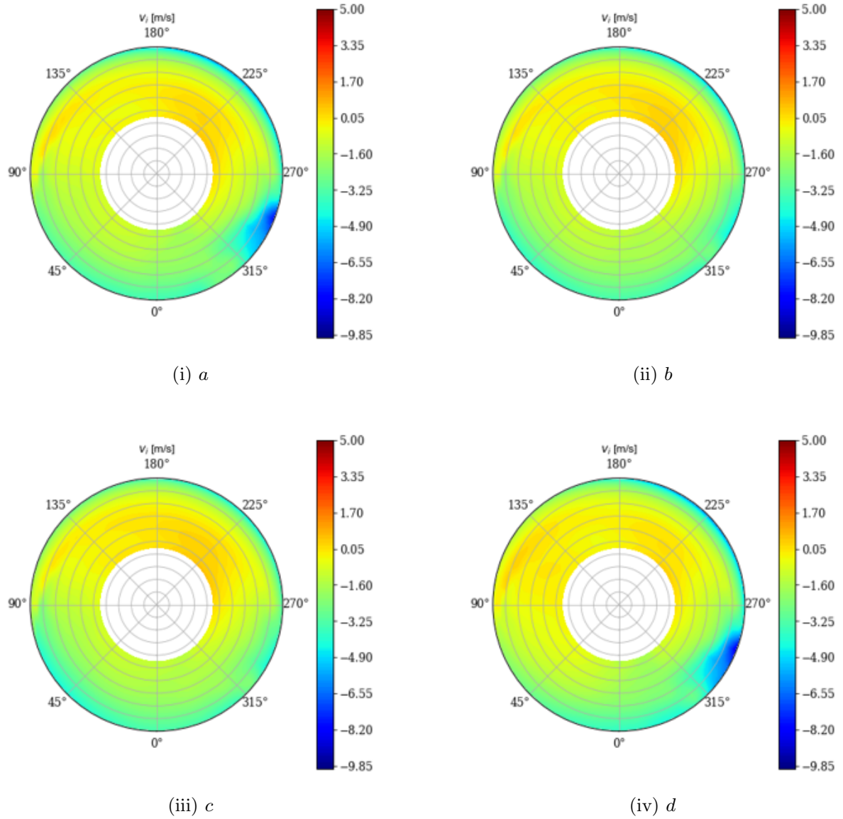
Fig.3.5: 誘導速度 v_i の分布
