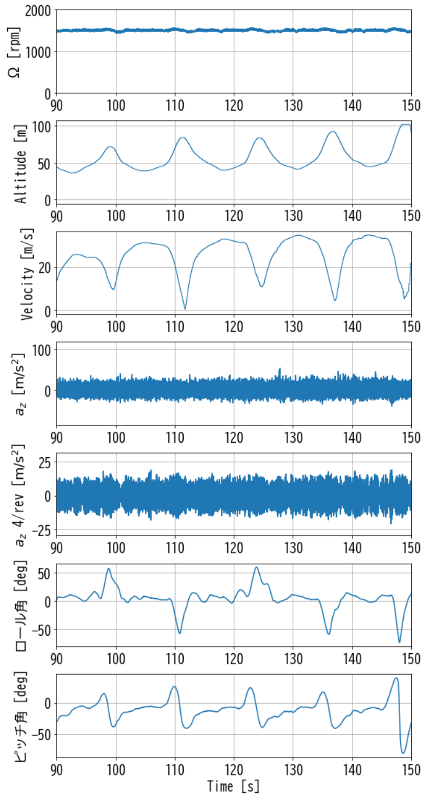
Fig.2.6: 飛行試験の各データ (case a )
