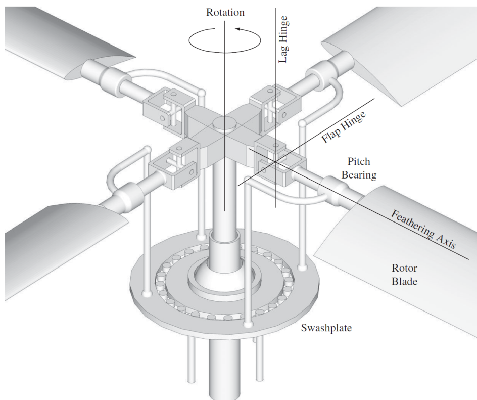
Fig.2.2: 関節式ローターハブと根元の概略図 [12]
