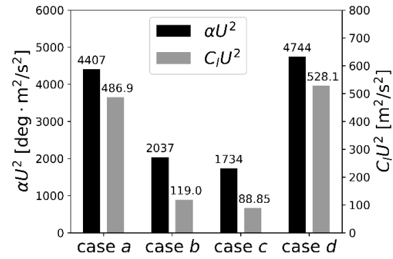
Fig.3.18: \alpha U^2, C_l U^2 の振幅 (product 5)
