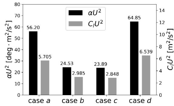
Fig.3.16: \alpha U^2, C_l U^2 の振幅 (product 3)
