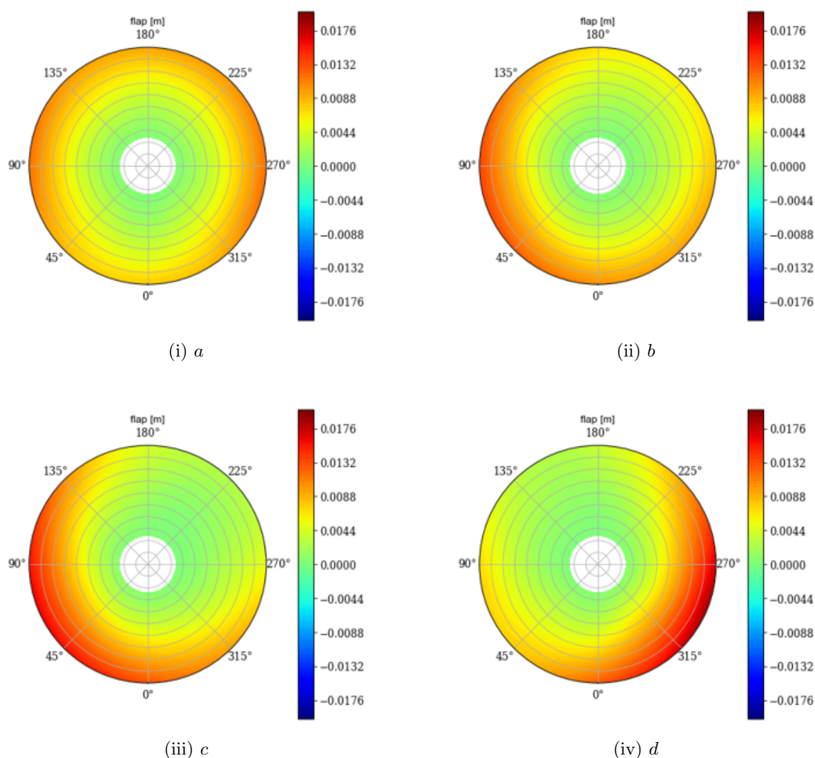
Fig.3.9: フラップの分布
