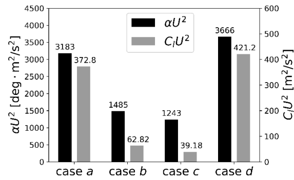
Fig.3.19: \alpha U^2, C_l U^2 の振幅
