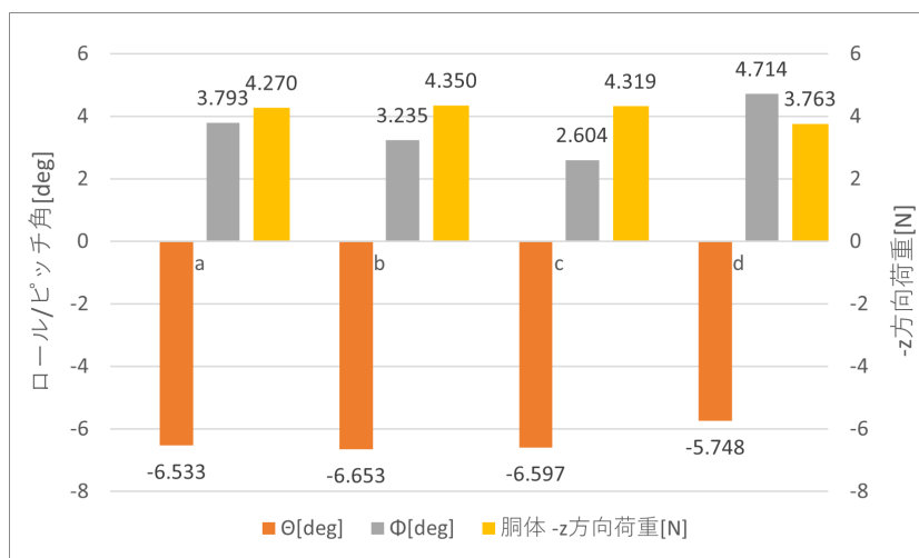
Fig.3.21: 機体ロール/ピッチ角および胴体 -z 方向荷重
