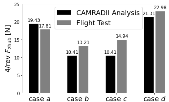
Fig.3.1: CAMRAD II と飛行試験の F_{z\text{hub}} の比較
