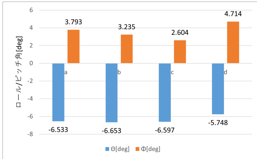
Fig.3.6: 機体の姿勢角
