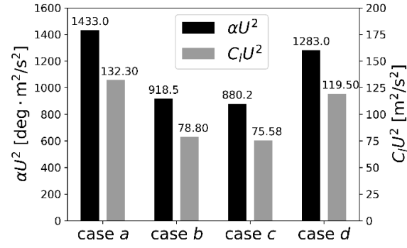
Fig.3.17: \alpha U^2, C_l U^2 の振幅 (product 4)
