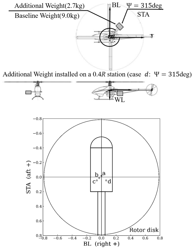
Fig.2.3: 飛行試験用ラジコンヘリコプタと錘取り付け位置
