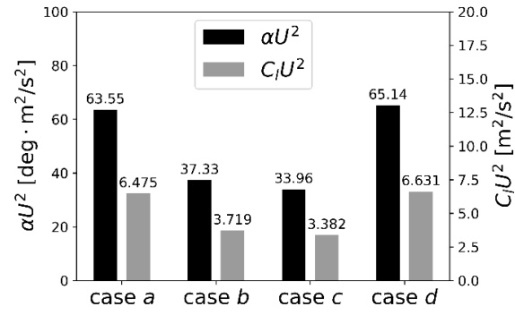
Fig.3.15: \alpha U^2, C_l U^2 の振幅 (product 2)
