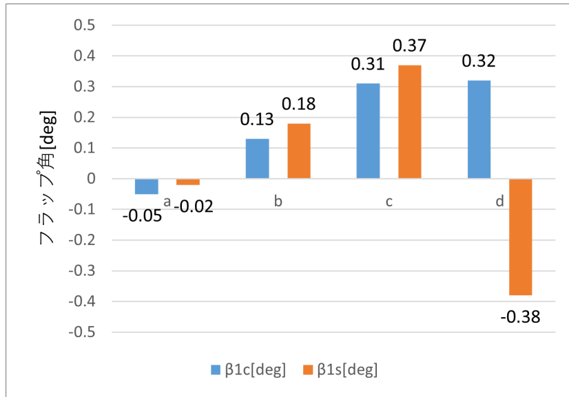
Fig.3.10: フラップ角
