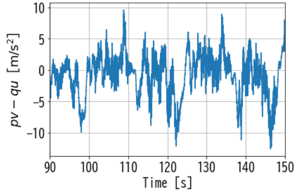
Fig.3.2: 飛行試験の pv - qu (case a )
