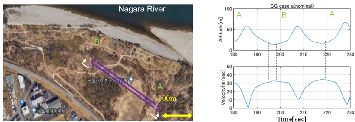
Fig.2.5: 飛行試験場と高度, 速度のデータ
