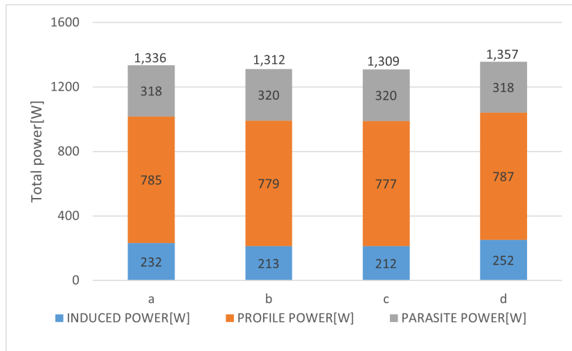
Fig.3.20: メインロータの必要パワーの比較
