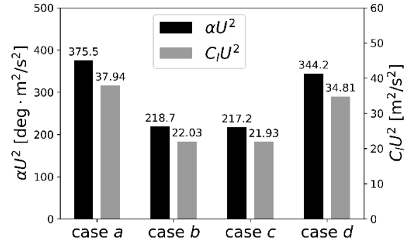
Fig.3.14: \alpha U^2, C_l U^2 の振幅 (product 1)
