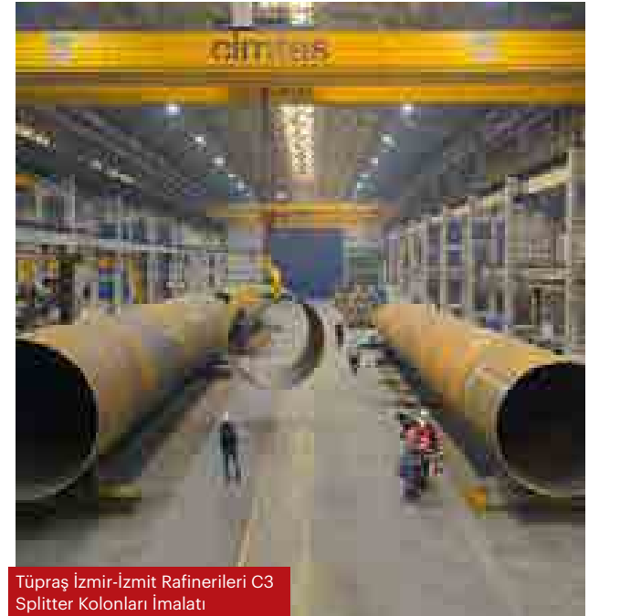
Tüpraş İzmir-İzmit Rafinerileri C3 Splitter Kolonları Gövde İmalatı
