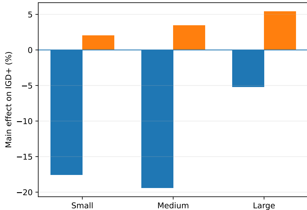
IGD+
