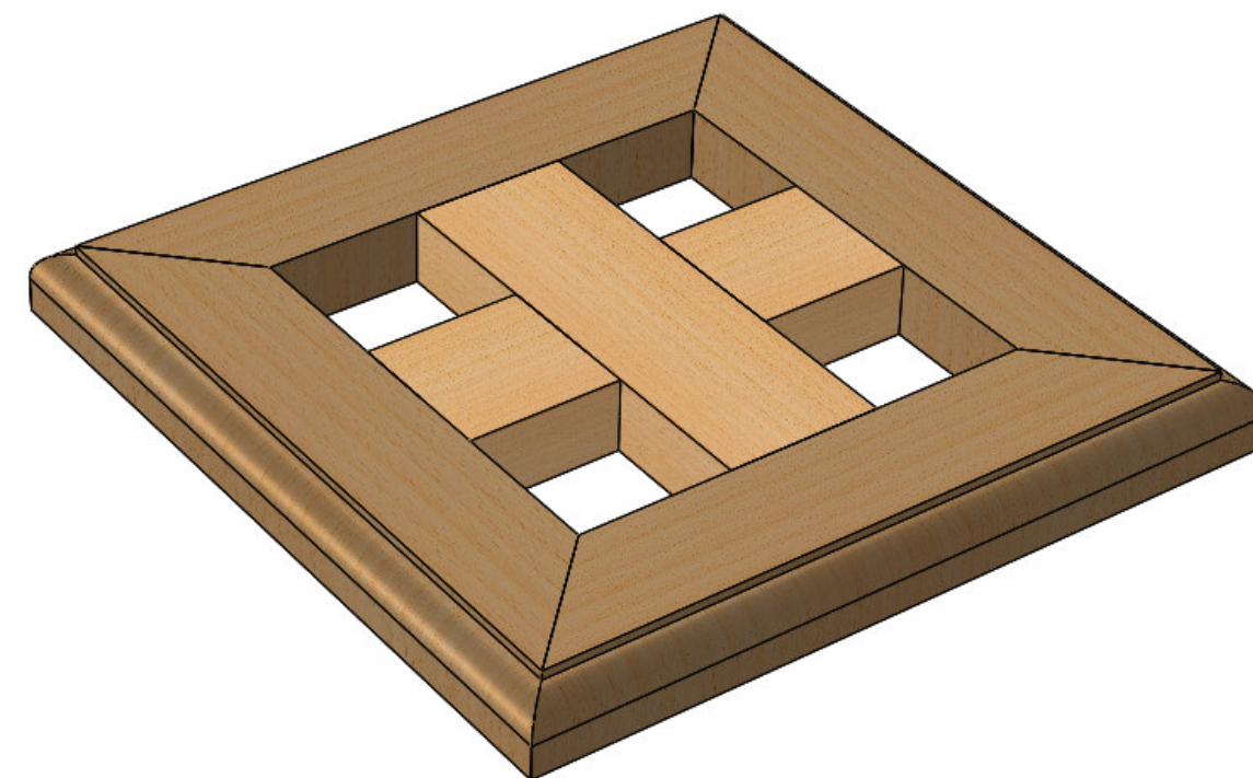
Assemblage DOMINO
