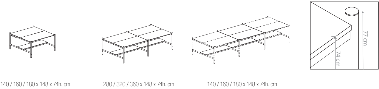
140 / 160 / 180 x 148 x 74h. cm 280 / 320 / 360 x 148 x 74h. cm 140 / 160 / 180 x 148 x 74h. cm
