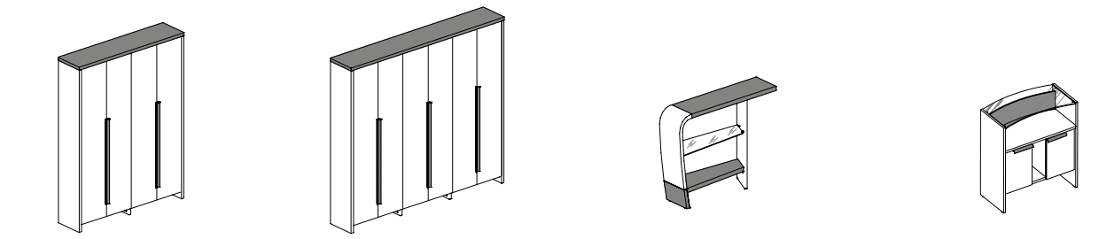
L.188cm P.45cm H.209cm L.278cm P.45cm H.209cm L.140cm P.34cm H.95cm L.130cm P.60cm H.110cm
