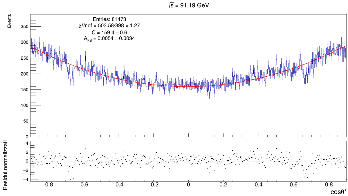
Figura 4: Simulazione del canale muonico e^+e^- \rightarrow \mu^+\mu^- .
