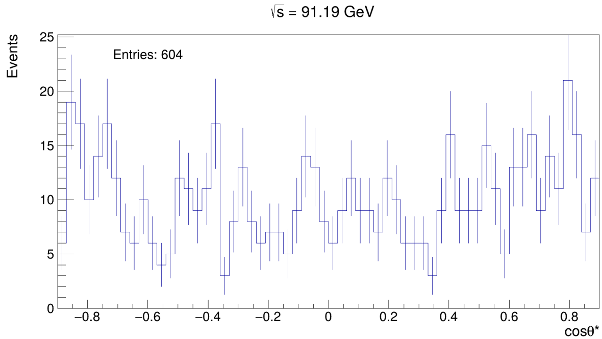
Figura 5: Simulazione del background del canale tau e^+e^- \rightarrow \tau^+\tau^- , dopo i tagli applicati, numero di eventi iniziali 99110.
