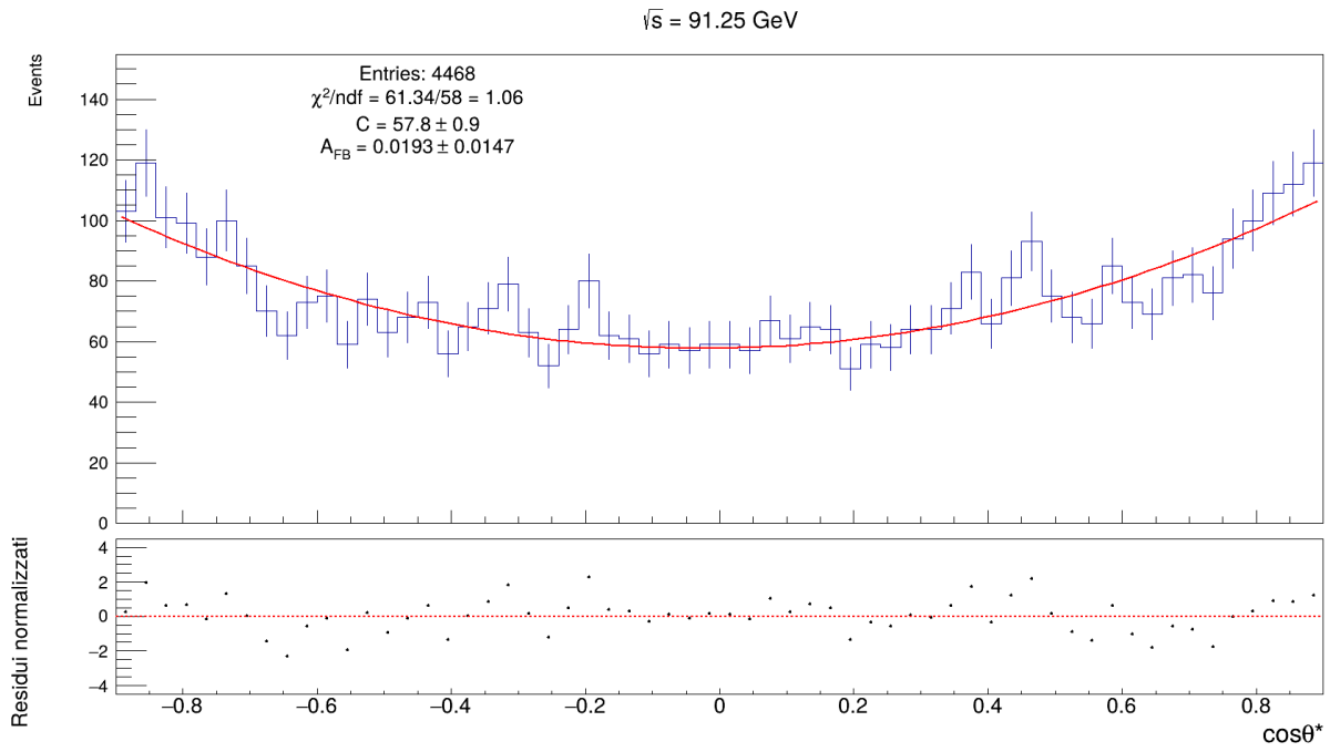
Figura 2: Distribuzione angolare e fit a \sqrt{s} = 91.25 \text{ GeV} .
