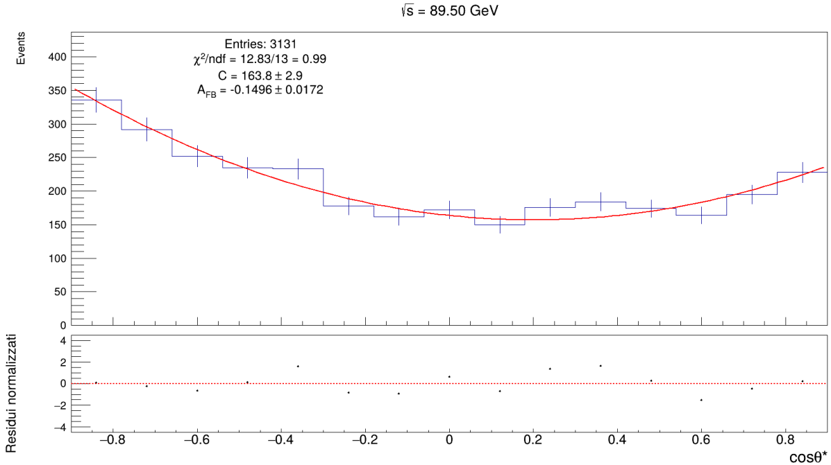
Figura 1: Distribuzione angolare e fit a \sqrt{s} = 89.50 GeV.
