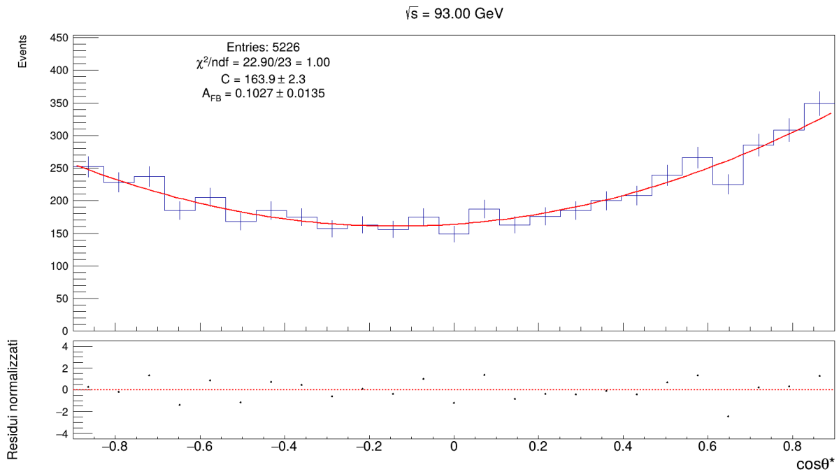
Figura 3: Distribuzione angolare e fit a \sqrt{s} = 93.00 \text{ GeV} .
