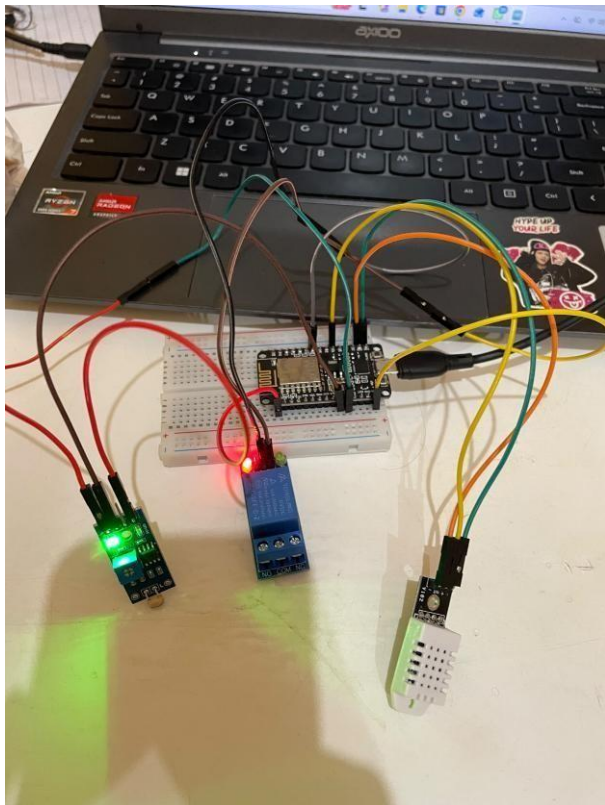
Contoh kondisi buruk output dan perangkat akuatornya
