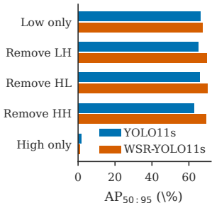
(b) Haar ablation
