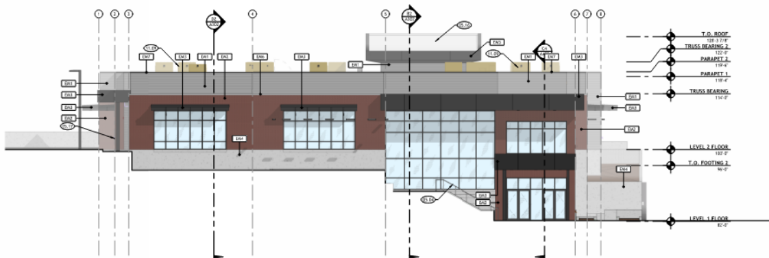
D1 WEST ELEVATION ASST SCALE: 1/8" = 1'-0"
