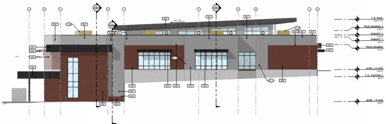
D1 SOUTH ELEVATION A201 SCALE: 1/8" = 1'-0"
