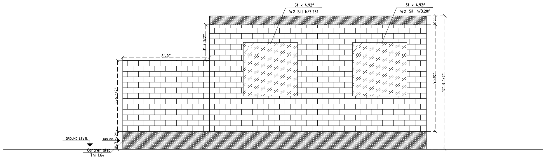
RIGHT ELEVATION
