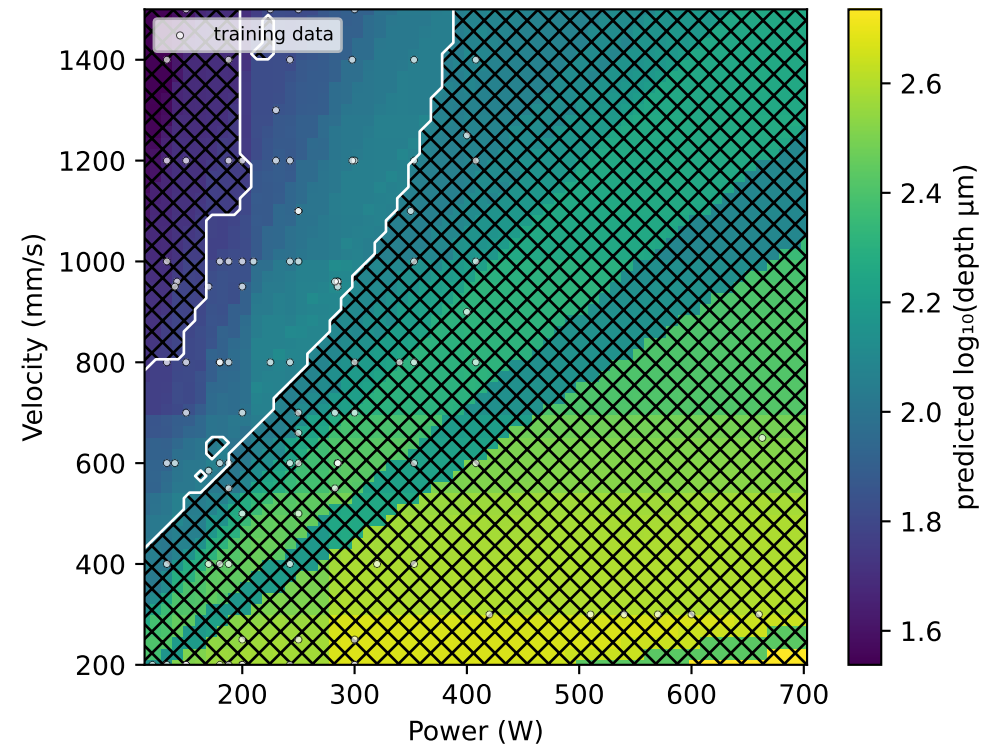
IN718 (n=127)
