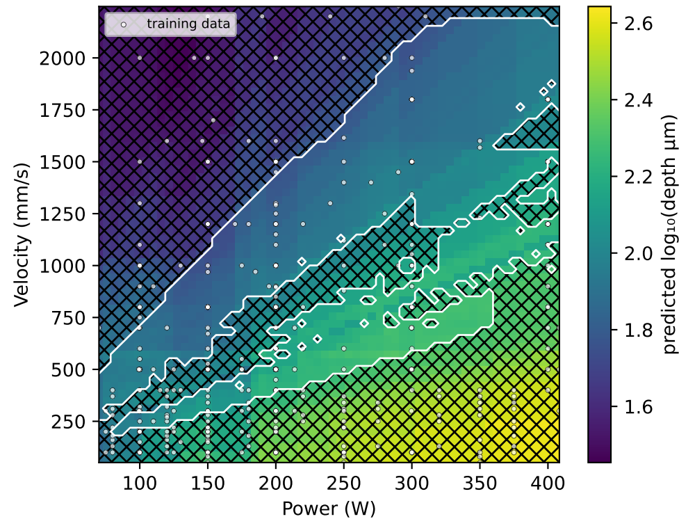
SS316L (n=382)
