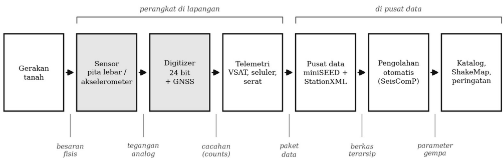
Gambar 2.9. Rantai akuisisi data seismik digital modern, dari gerakan tanah sampai basis data dan pengguna.
