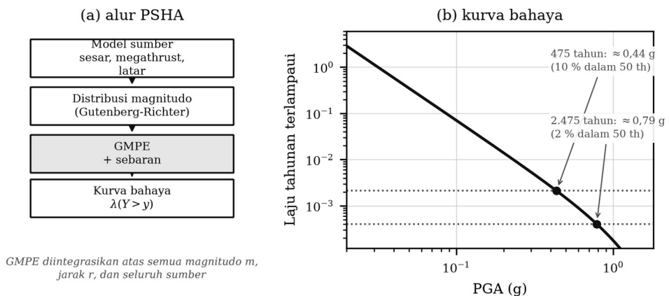
Gambar 10.1. (a) Skema alur PSHA dari model sumber, distribusi magnitudo, dan GMPE menuju kurva bahaya. (b) Contoh kurva bahaya dengan penandaan periode ulang 475 dan 2.475 tahun.
