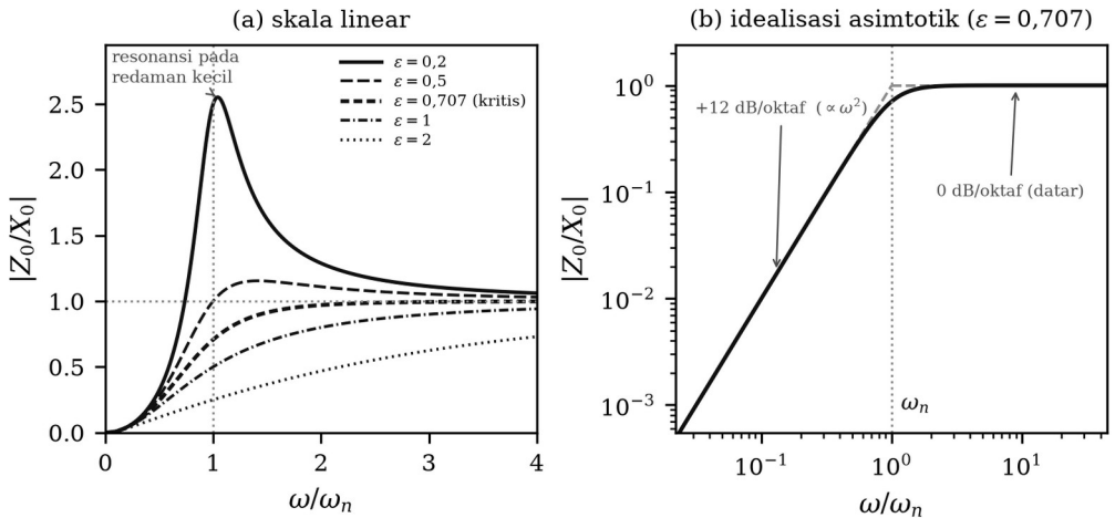
Gambar 2.5. Tanggapan amplitudo seismometer sebagai fungsi frekuensi sudut (kiri) dan idealisasi asimtotiknya dalam skala logaritmik (kanan). Angka pada gambar kanan menunjukkan kemiringan garis dalam dB/oktaf.
