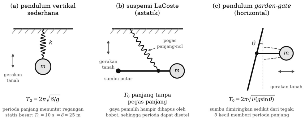
Gambar 2.8. Perubahan konfigurasi sistem massa-pegas untuk memperpanjang perioda natural: (a) pendulum vertikal sederhana, (b) suspensi LaCoste dengan pegas panjang-nol, (c) pendulum garden-gate untuk komponen horizontal.
