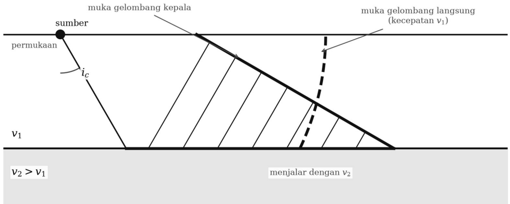
Gambar 3.5. Penjalaran gelombang kepala dan proses kejadiannya menurut asas Huygens.
