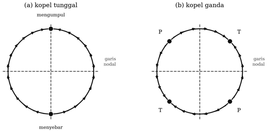
Gambar 5.13. Arah polarisasi gelombang S di permukaan bola fokus untuk sumber (a) kopel tunggal dan (b) kopel ganda.
