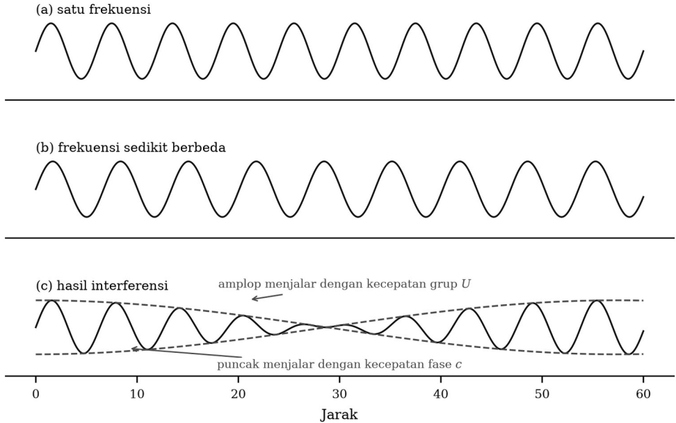
Gambar 3.11. Ilustrasi kecepatan fase dan kecepatan grup: (a) gelombang sinus berfrekuensi tunggal, (b) gelombang sinus dengan frekuensi sedikit berbeda, dan (c) hasil interferensi keduanya. Amplop (c) menjalar dengan kecepatan grup.
