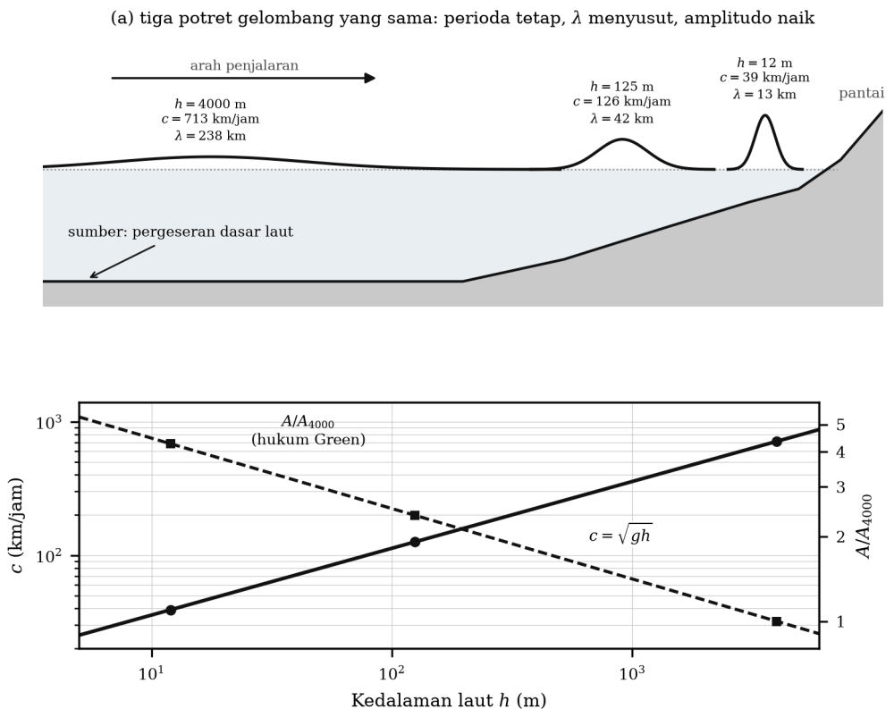
Gambar 11.1. Penjalaran tsunami dari sumber di zona subduksi menuju pantai: perubahan kecepatan, panjang gelombang, dan tinggi gelombang akibat pendangkalan.
