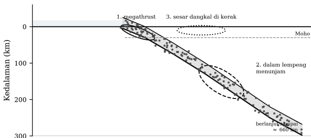
Gambar 7.3. Skema penampang zona Wadati-Benioff pada busur Sunda dengan tiga kelompok sumber gempa: megathrust, dalam lempeng menunjam, dan sesar dangkal di kerak atas.
