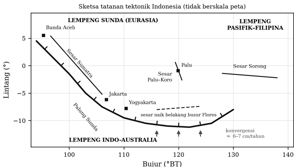
Gambar 7.1. Sketsa tatanan tektonik Indonesia: palung, arah dan laju konvergensi lempeng, serta jalur sesar aktif utama. Sketsa skematis; untuk kerja kuantitatif gunakan peta sumber gempa resmi.
