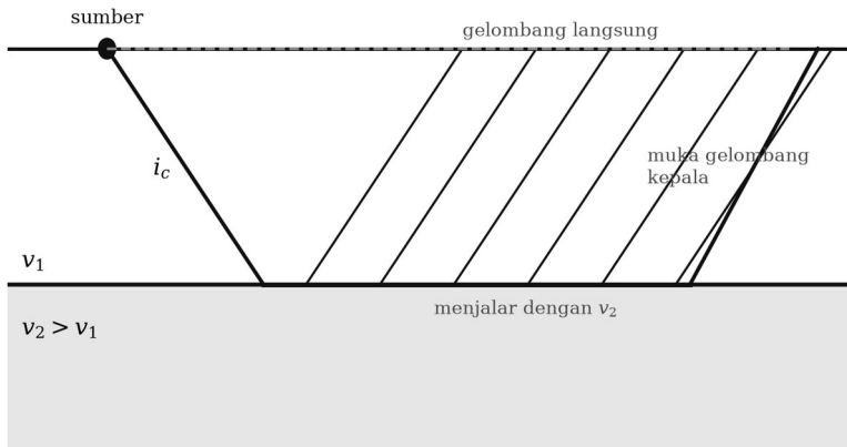
Gambar 3.5. Penjalaran gelombang kepala dan proses terjadiannya menurut asas Huygens.
