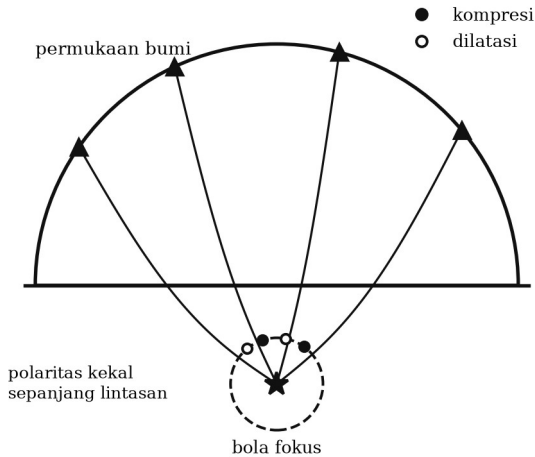
Gambar 5.3. Polaritas gerakan pertama gelombang P yang kekal sepanjang penjalarannya memungkinkan polaritas di bola fokus disimpulkan dari pengamatan di permukaan bumi.
