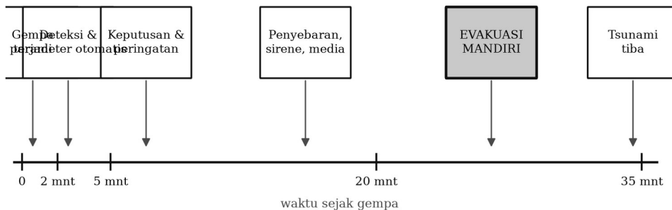
Gambar 11.2. Alur kerja peringatan dini tsunami: dari deteksi gelombang P, penentuan parameter, pencocokan skenario, sampai penyebaran peringatan dan evakuasi. Sumbu waktu menunjukkan mengapa “rantai terakhir” sering menjadi yang paling menentukan.
