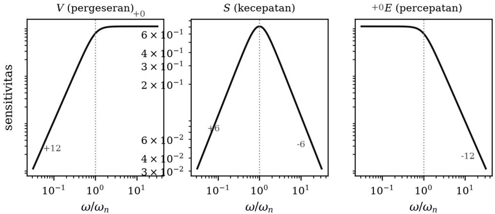
Gambar 2.6. Sensitivitas pergeseran V , kecepatan S , dan percepatan E untuk seismometer mekanis. Angka dalam gambar menyatakan kemiringan asimtot dalam dB/oktaf.
