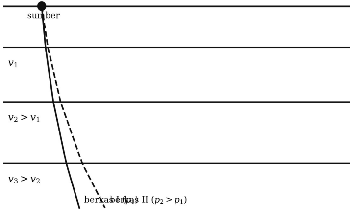
Gambar 3.3. Penjalaran dua berkas gelombang dengan parameter gelombang yang berbeda pada medium tiga lapis. Berkas dengan p lebih besar berjalan lebih landai dan menembus lebih dangkal.
