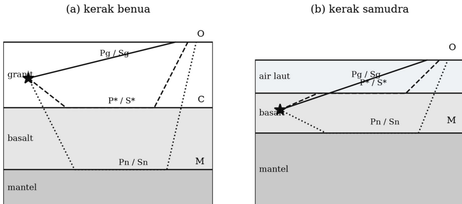
Gambar 3.9. Struktur kerak bumi, fase gelombang, dan penjalarnya untuk (a) kerak benua dan (b) kerak samudra. Digambar ulang mengikuti Båth (1979).
