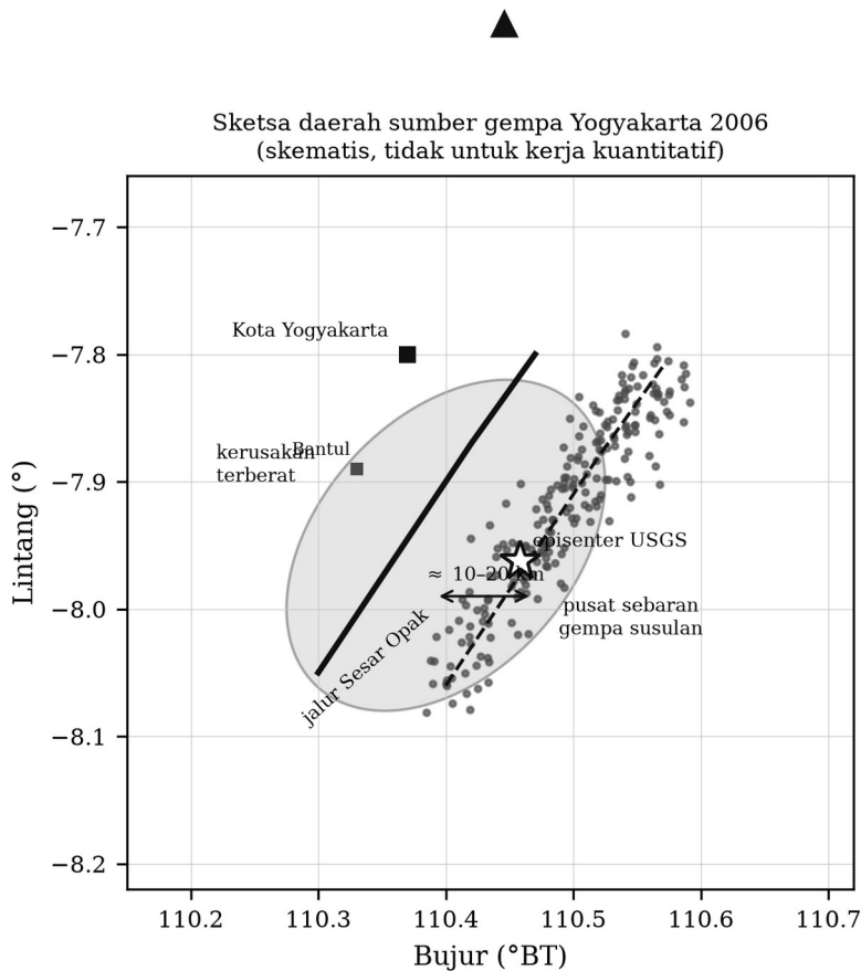
Gambar 14.1. Sketsa daerah sumber gempa Yogyakarta 2006: posisi episenter instrumental, jalur Sesar Opak, daerah pusat sebaran gempa susulan yang
