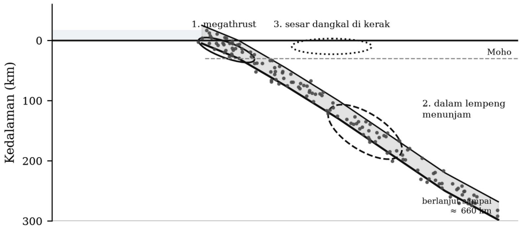
Gambar 7.2. Skema penampang zona Wadati-Benioff pada busur Sunda dengan tiga kelompok sumber gempa: megathrust, dalam lempeng menunjam, dan sesar dangkal di kerak atas.
