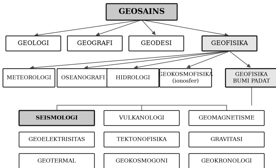
Gambar 1.1. Pembagian geosains, geofisika, dan geofisika bumi padat. Batas antarcabang bersifat administratif belaka; dalam praktik penelitian modern hampir semua persoalan penting dikerjakan lintas cabang.
