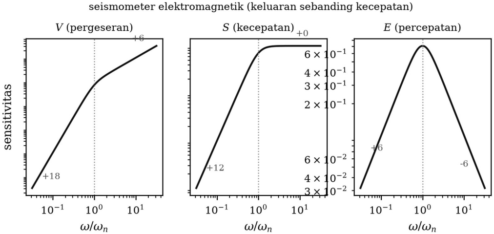
Gambar 2.7. Sensitivitas pergeseran, kecepatan, dan percepatan untuk seismometer elektromagnetik.
