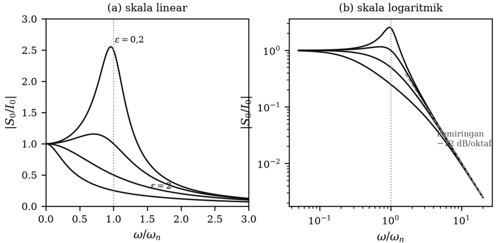
Gambar 2.3. Tanggapan amplitudo sistem orde dua: (a) dengan skala linear, dan (b) dengan skala logaritmik, untuk beberapa harga faktor redaman \varepsilon .
