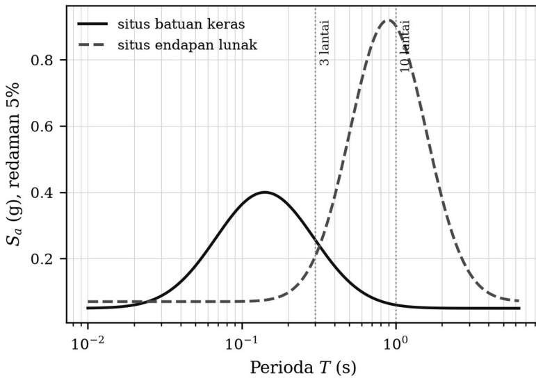
Gambar 9.1. Spektrum tanggapan percepatan untuk redaman 5 persen: kurva tanah keras dibandingkan dengan tanah lunak. Puncak spektrum tanah lunak bergeser ke perioda yang lebih panjang dan bernilai jauh lebih besar.
