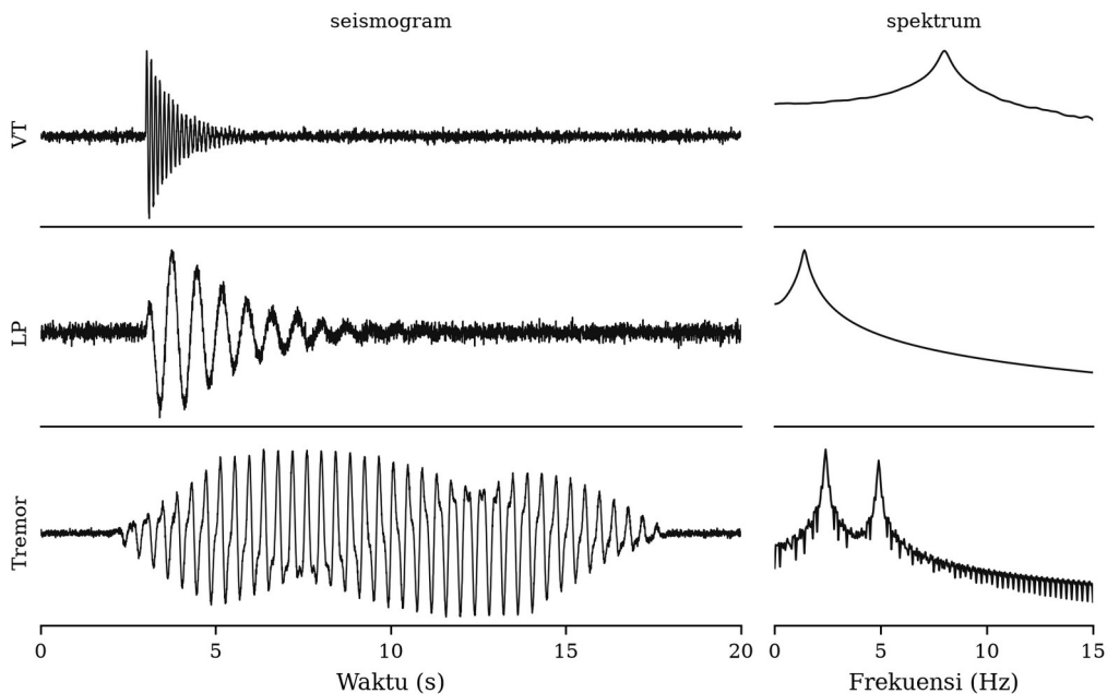
Gambar 12.1. Seismogram dan spektrum skematis untuk gempa VT, LP, dan tremor vulkanik. Perhatikan perbedaan ketajaman awal sinyal dan kandungan frekuensinya.
