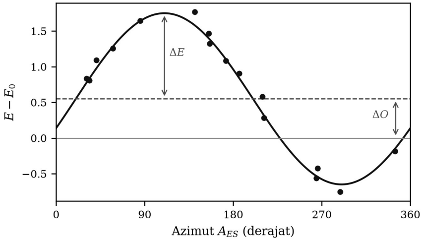
Gambar 4.4. Grafik E - E_0 terhadap azimuth A_{ES} pada metode Richter. Pergeseran vertikal rata-rata menentukan koreksi waktu kejadian, sedangkan amplitudo dan fase sinusnya menentukan koreksi posisi episenter.
