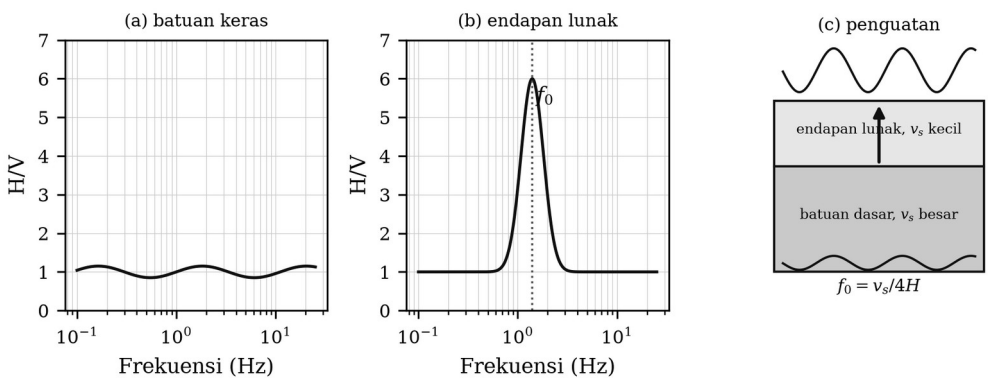
Gambar 9.2. Kurva HVS khas: (a) situs batuan keras, tanpa puncak jelas; (b) situs endapan lunak, dengan puncak tajam pada frekuensi dasar f_0 ; (c) skema penguatan gelombang pada lapisan lunak di atas batuan dasar.
