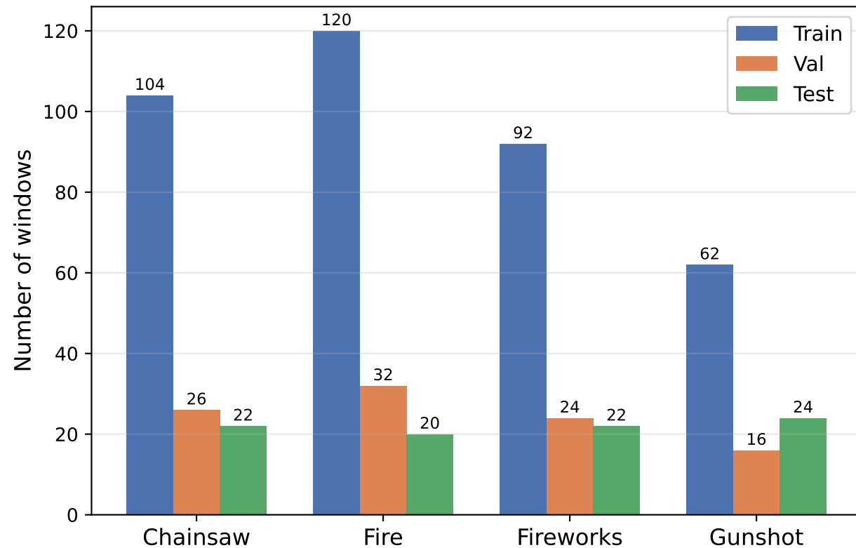
Dataset windows per class (best config: N_{mel}=32 , N_{fr}=32 )
