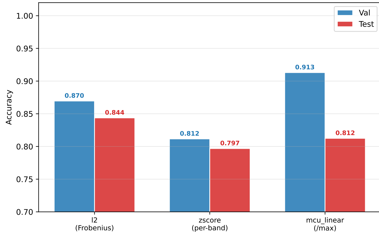
mel20×fr38
