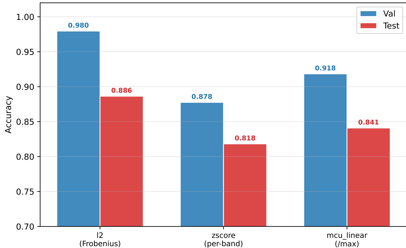
mel32×fr32
