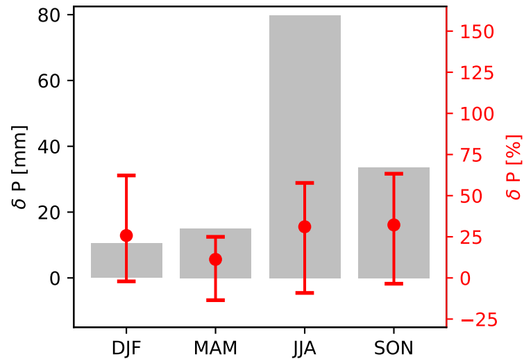
AWI-ESM-1-1-LR
