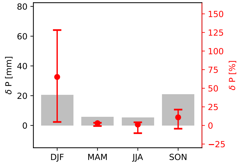
MIROC-ES2L
