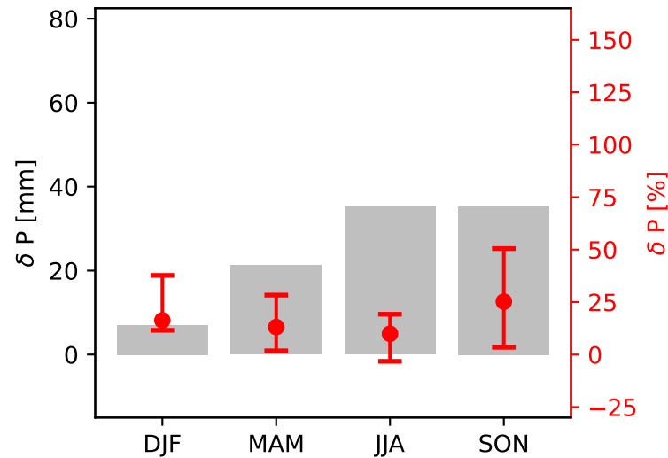
MPI-ESM1-2-LR
