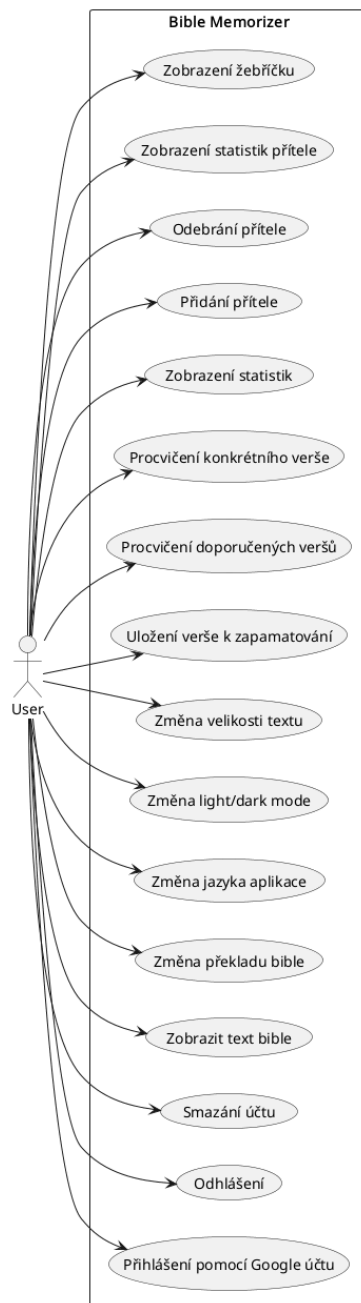
Obrázek 8: Use Case diagram aplikace
