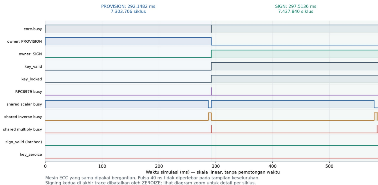
Gambar 1. Trace RTL pada 25 MHz: provisioning, signing, lalu signing kedua yang dibatalkan dengan ZEROIZE. Sumbu waktu linear; pulsa satu siklus (40 ns) tampak tipis pada skala ms. Detail tahap dan handshake terdapat pada lampiran.
