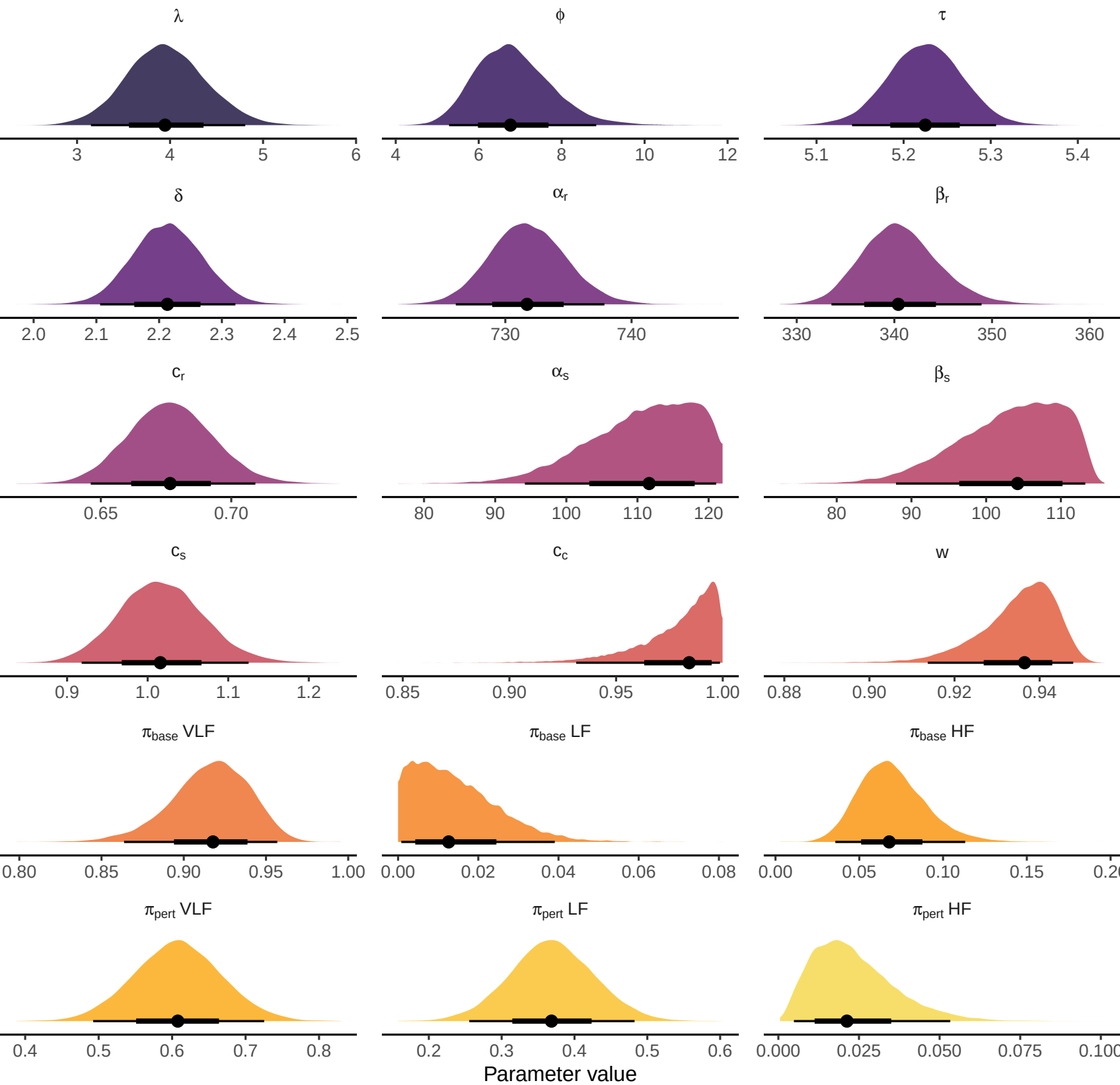
Posterior distribution of model parameters
