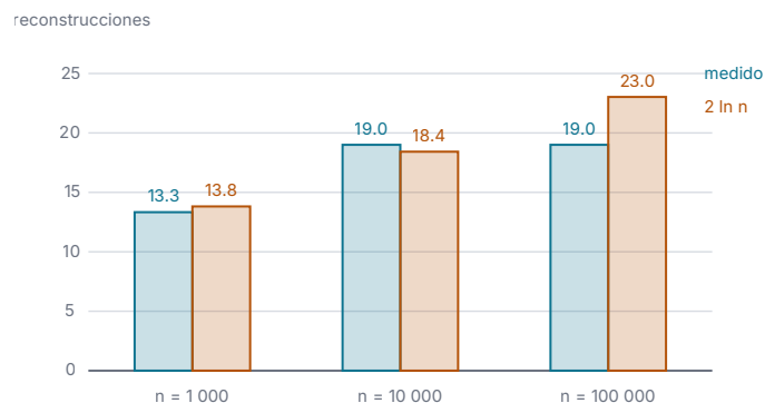
Figura 11. Lo que predice el análisis hacia atrás y lo que reconstruye el programa.
