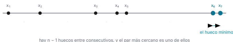
Figura 3. Ordenados, solo quedan n - 1 huecos que mirar.
