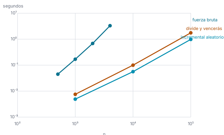
Figura 12. Los tres algoritmos de la clase, en ejes logarítmicos, con los tiempos que este documento acaba de medir. La pendiente es el exponente: 2 para la fuerza bruta, 1 para los otros dos.
