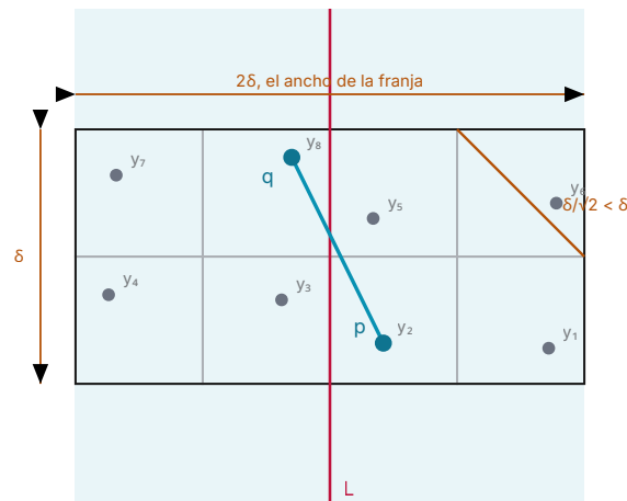
Figura 5. El rectángulo R partido en ocho cuadrados de lado \delta/2 . Cada cuadrado está entero de un lado de L y aguanta a lo sumo un punto, así que R aguanta ocho. Los puntos van numerados por su posición en el orden de y .
