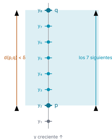
Figura 6. Los mismos ocho puntos, vistos solo como orden de y . Es la configuración extrema: q es el último punto que p tiene que mirar.
