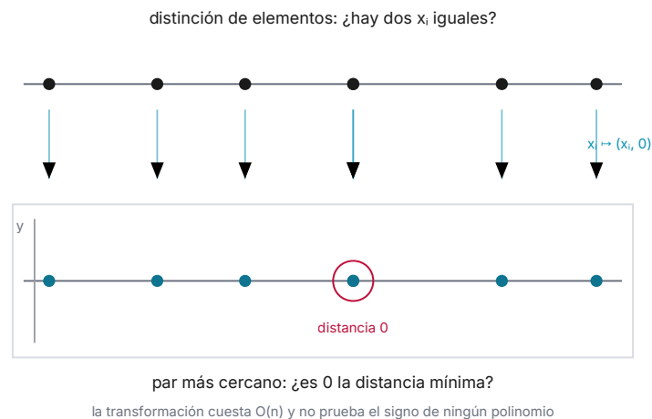
Figura 9. La reducción: los n reales se vuelven n puntos sobre el eje x . Dos valores iguales son dos puntos a distancia 0, así que la respuesta de un problema es la respuesta del otro.
