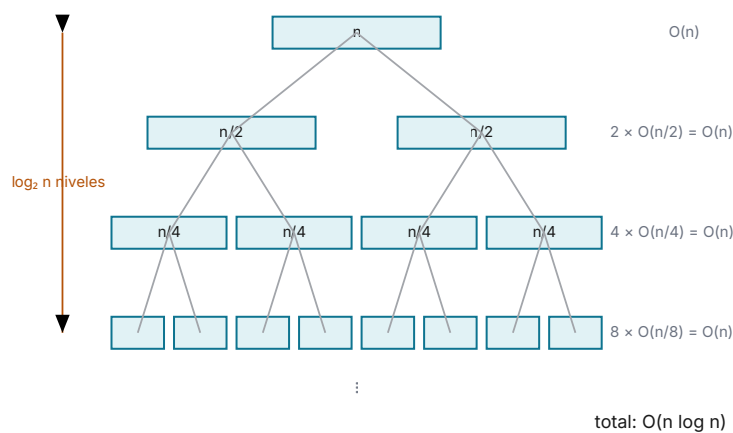
Figura 7. Repartir la lista ordenada por y cuesta O(n) por nivel, y hay \log_2 n niveles. Ordenar la franja en cada nivel costaría O(n \log n) por nivel, y ahí sale el logaritmo de más.
