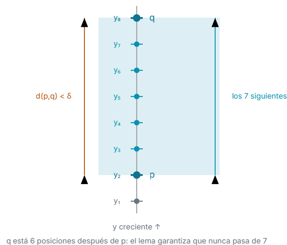
Figura 6. Los mismos ocho puntos, vistos solo como orden de y . Es la configuración extrema: q es el último punto que p tiene que mirar.
