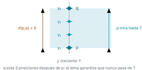
Figura 6. Los mismos puntos, vistos solo como orden de y . Aquí q está tres posiciones después de p . La demostración garantiza que nunca son más de siete.
