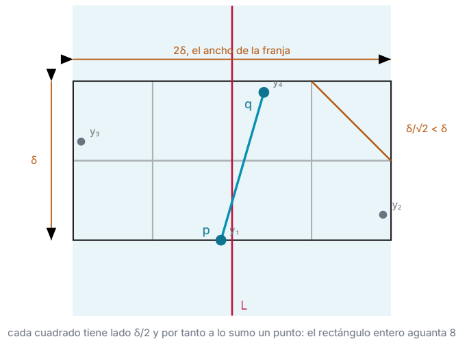
Figura 5. El rectángulo R partido en ocho cuadrados de lado \delta/2 . Cada cuadrado está entero de un lado de L y aguanta a lo sumo un punto, así que R aguanta a lo sumo ocho. Los cuatro puntos son una configuración posible: los del mismo lado están a distancia al menos \delta , y p y q a menos de \delta .
