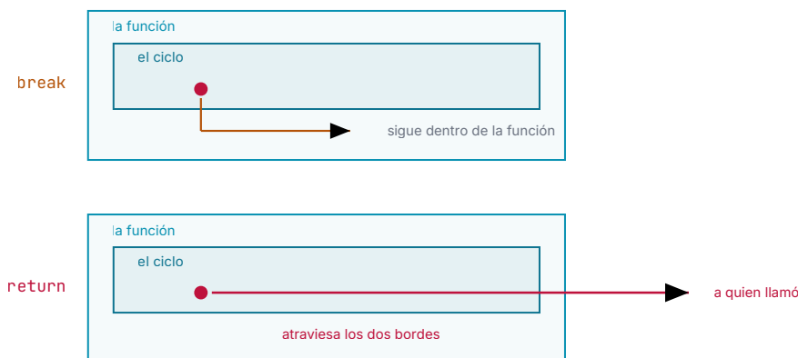
Figura 2. break termina el ciclo y el programa sigue dentro de la función. return atraviesa los dos bordes de una vez.
