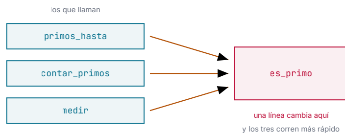
Figura 3. Ninguno de los tres sabe cómo se decide si un número es primo, así que la mejora se hace una vez y les llega a los tres.
