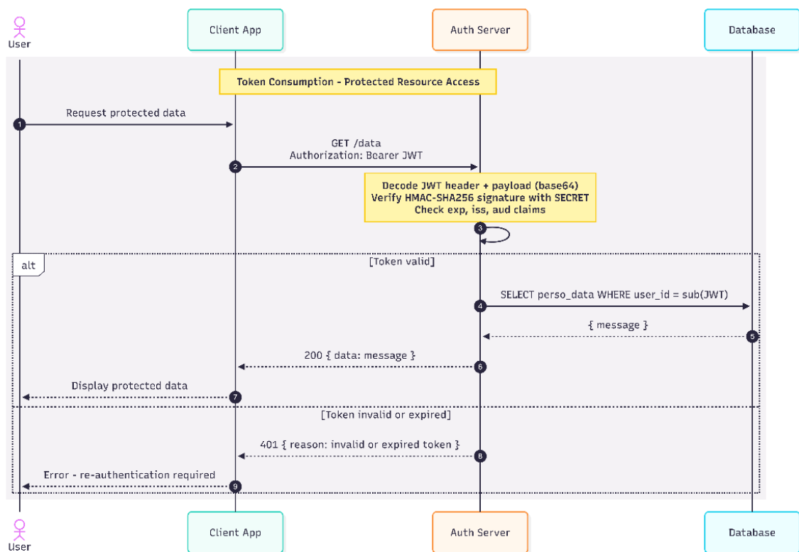
Figura 4. Consumul Token-ului
