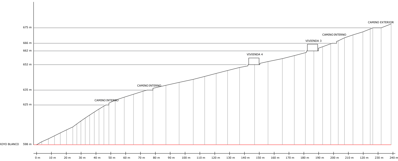
PERFIL DE CORTE 3
