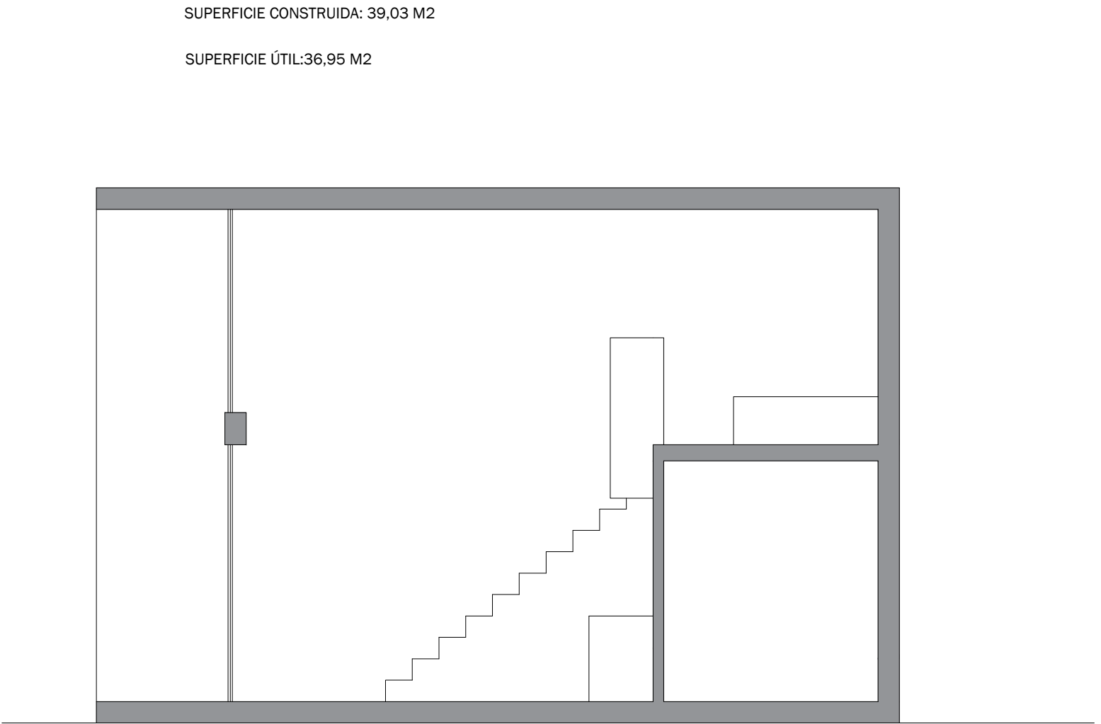
SECCIÓN PROTOTIPO ESCALA 1:50
