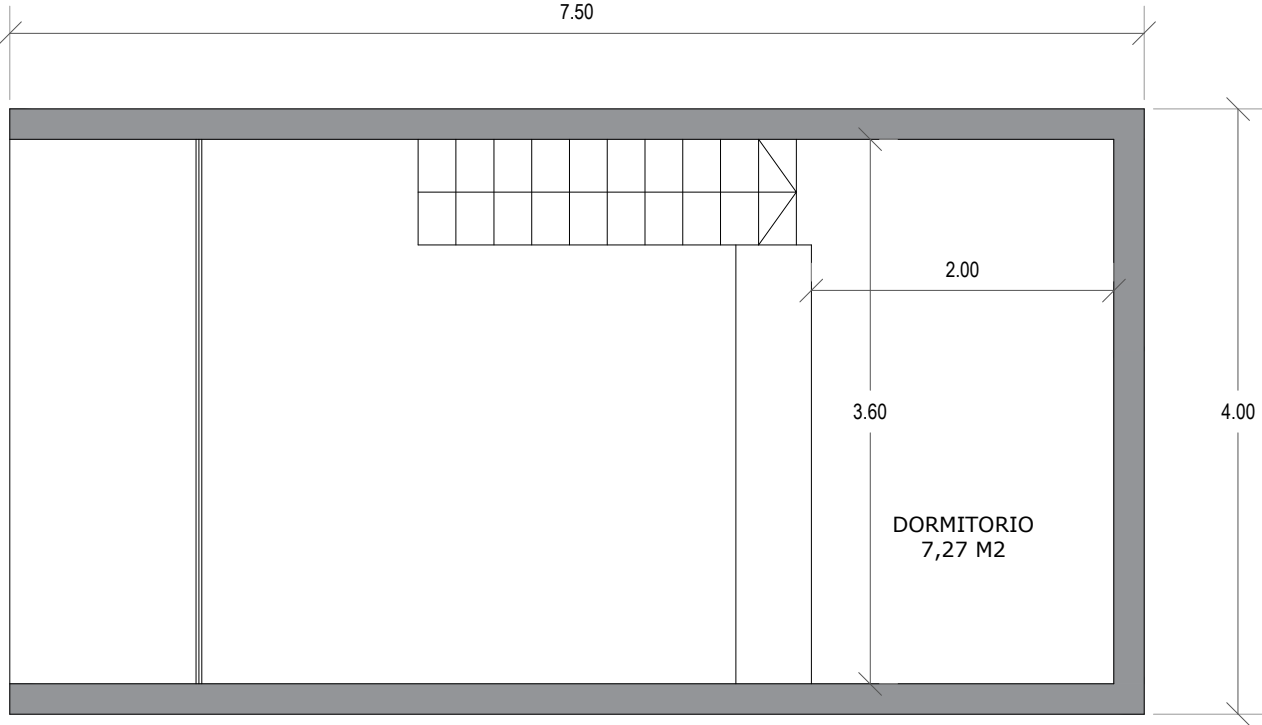
PLANTA ALTA PROTOTIPO ESCALA 1:50
