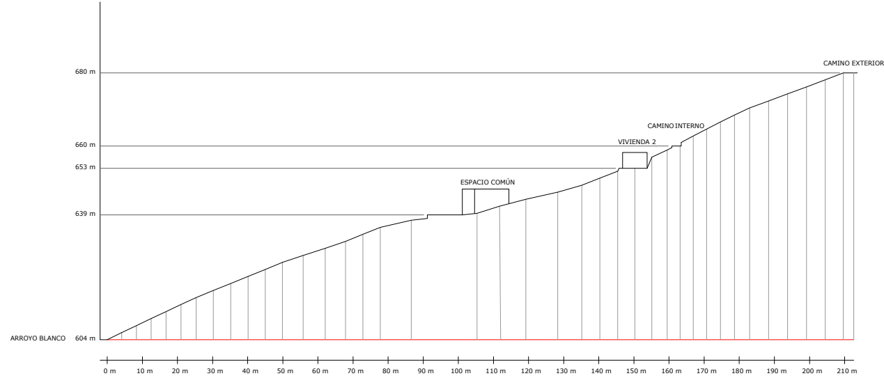
PERFIL DE CORTE 5
