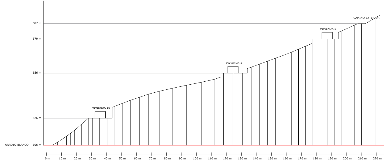
PERFIL DE CORTE 6
