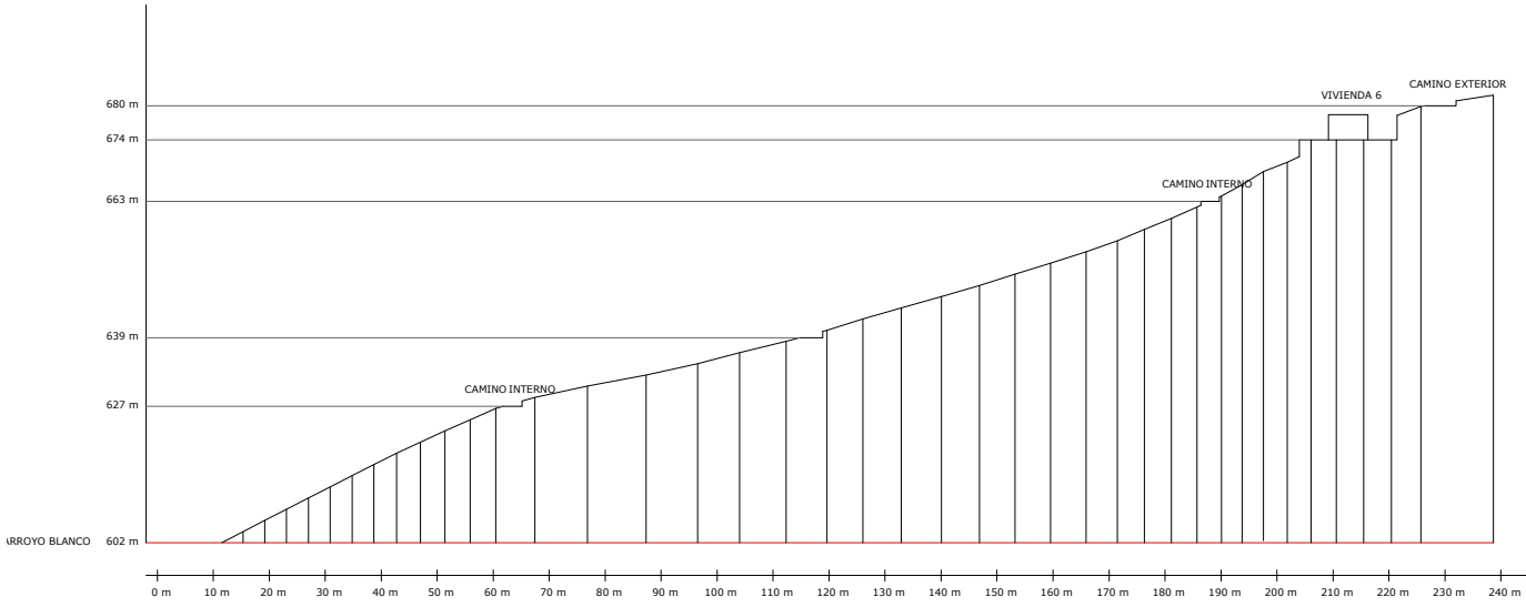
PERFIL DE CORTE 4
