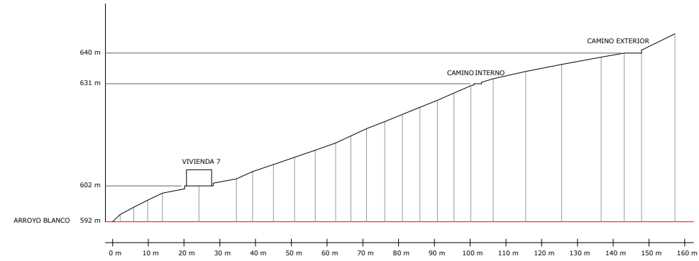
PERFIL DE CORTE 2
