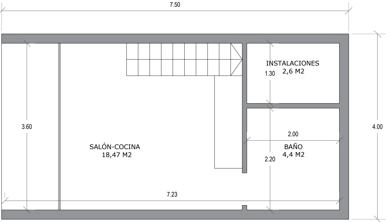
PLANTA BAJA PROTOTIPO ESCALA 1:50
