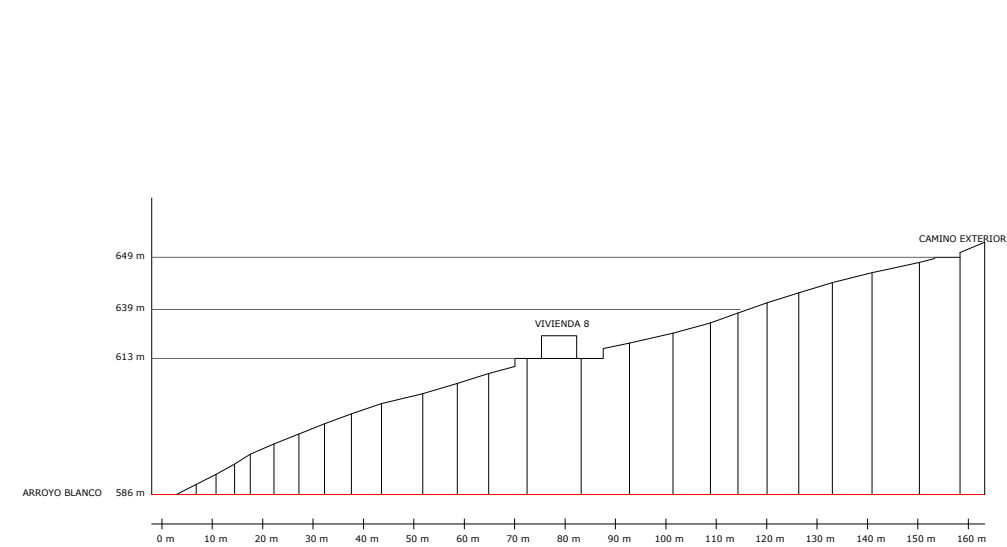
PERFIL DE CORTE 1
