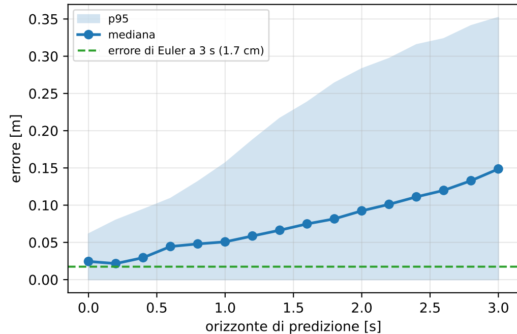
Errore di predizione contro l'impianto MuJoCo
