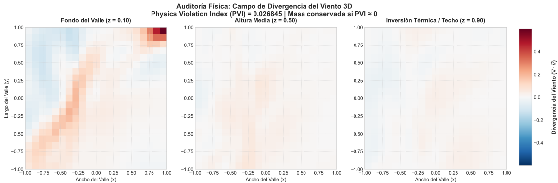
Figura 2: Cortes espaciales 2D de la divergencia del viento ( \nabla \cdot \vec{v} ) en tres alturas del Valle de Aburrá.
