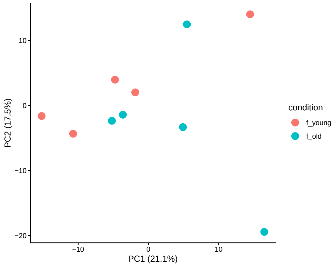
hisat2_PE DESeq2, top 500 genes
