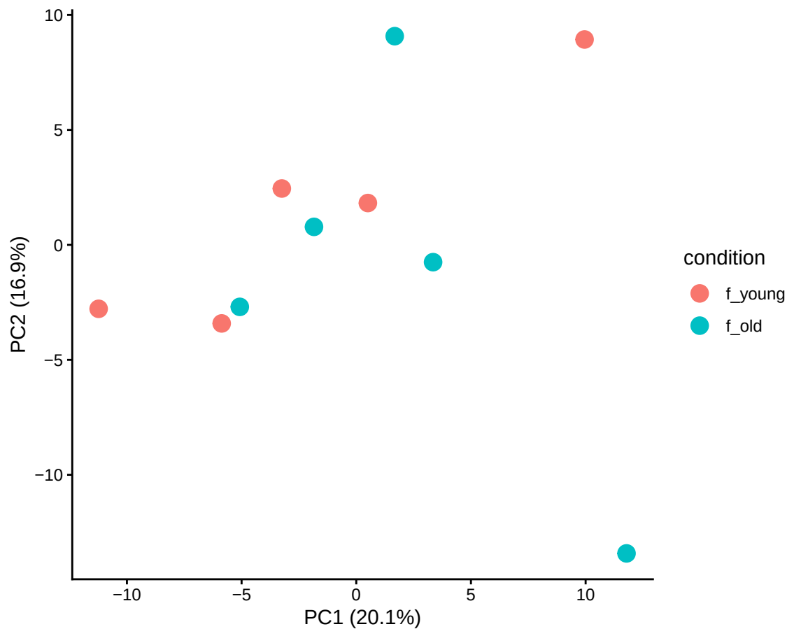
hisat2_PE DESeq2, top 250 genes
