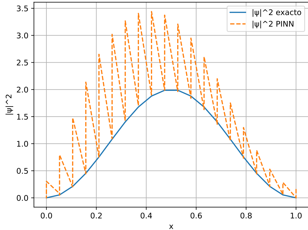
|\psi(x,T)|^2 en pozo infinito (n=1)
