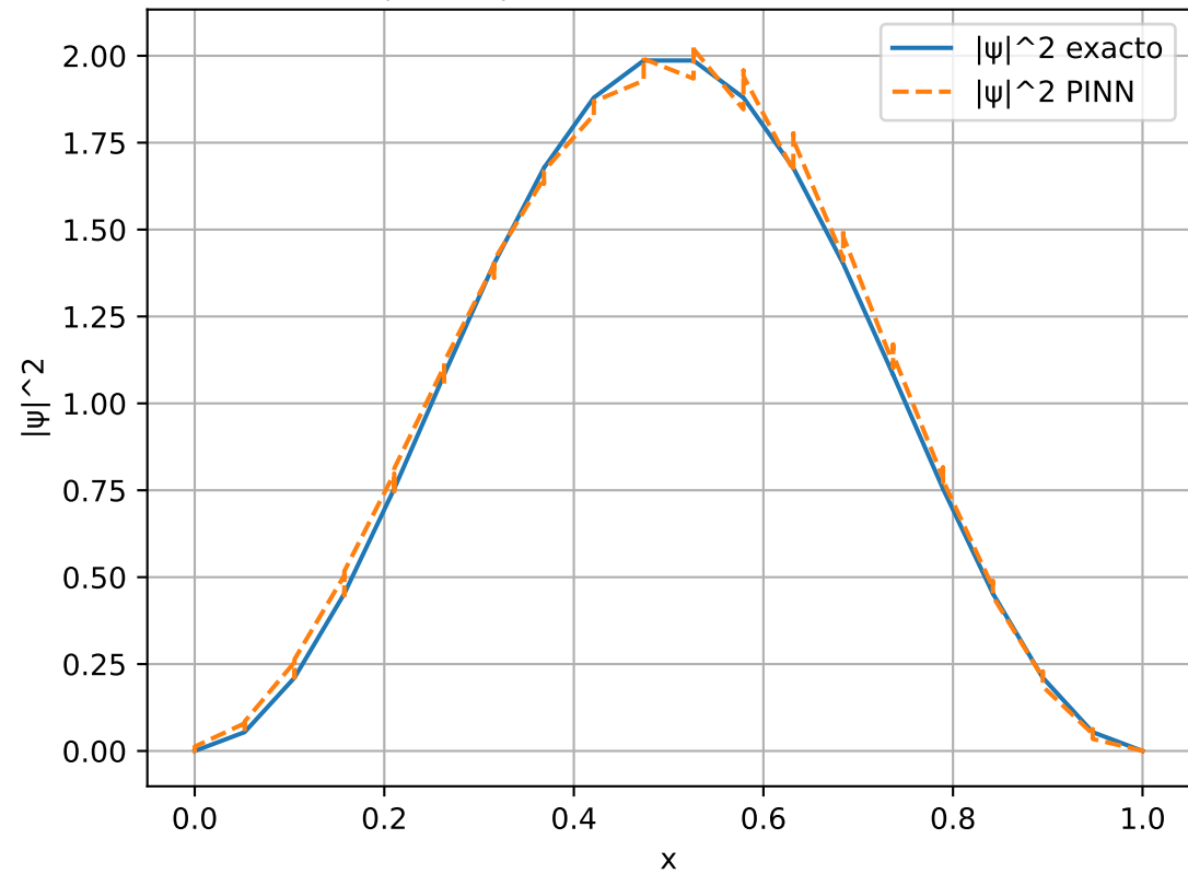
|\psi(x,T)|^2 en pozo infinito ( n=1 )
