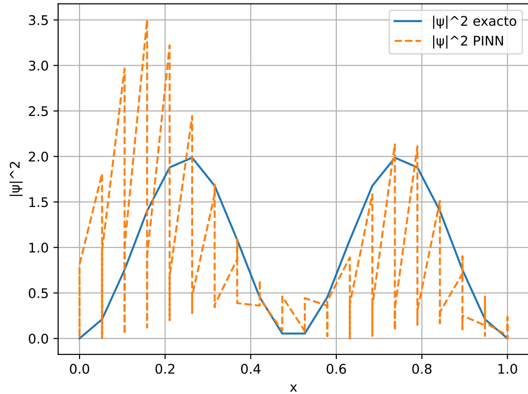
|\psi(x,T)|^2 en pozo infinito (n=2)
