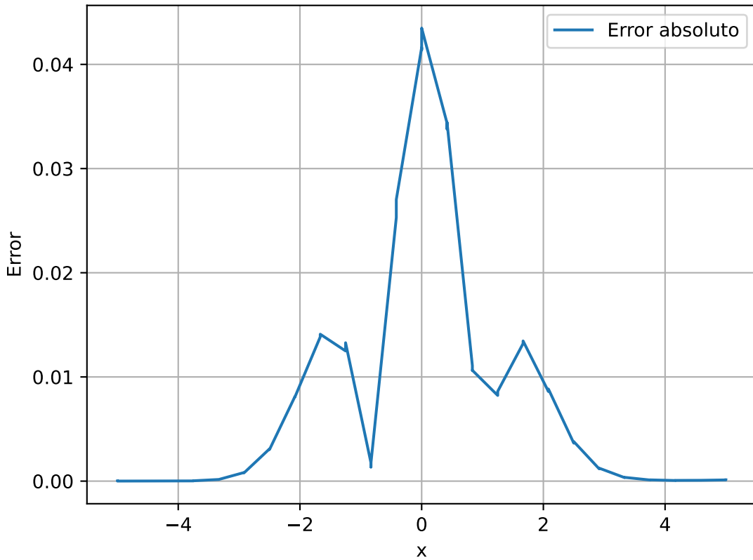
Error absoluto en |\psi(x,T)|^2
