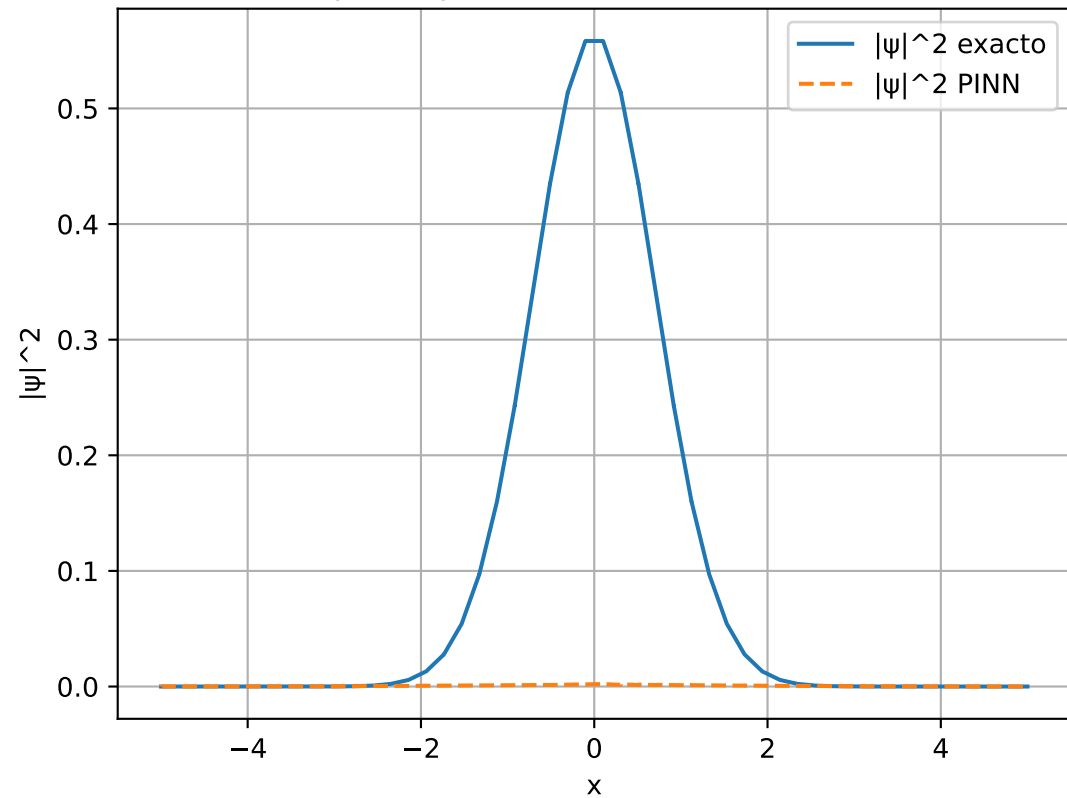
|\psi(x,T)|^2 en pozo infinito (n=0)
