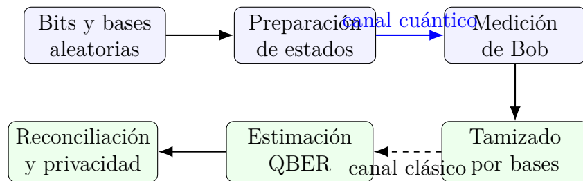
Figura 2.1: Secuencia funcional de BB84 desde preparación hasta postprocesamiento.
