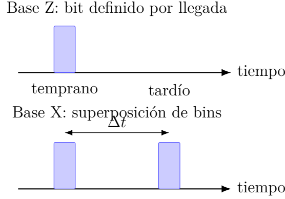
Figura 2.2: Representación esquemática de codificación time-bin .
