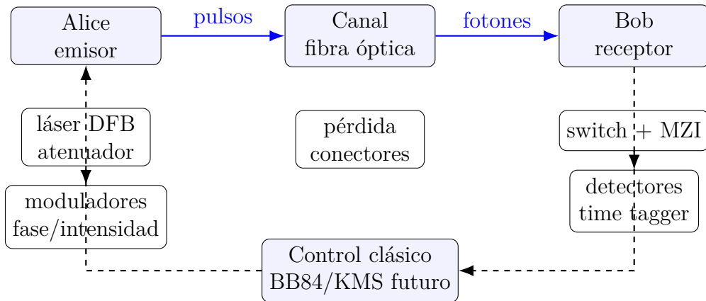
Figura 5.1: Bloques físicos de un enlace QKD time-bin .
