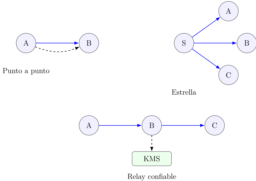
Figura 4.2: Topologías candidatas para una maqueta QKD de campus.
