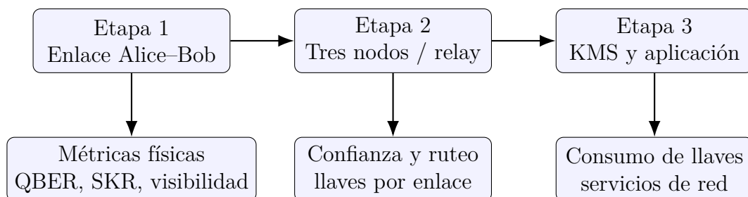
Figura 4.1: Evolución propuesta para una maqueta QKD de campus.
