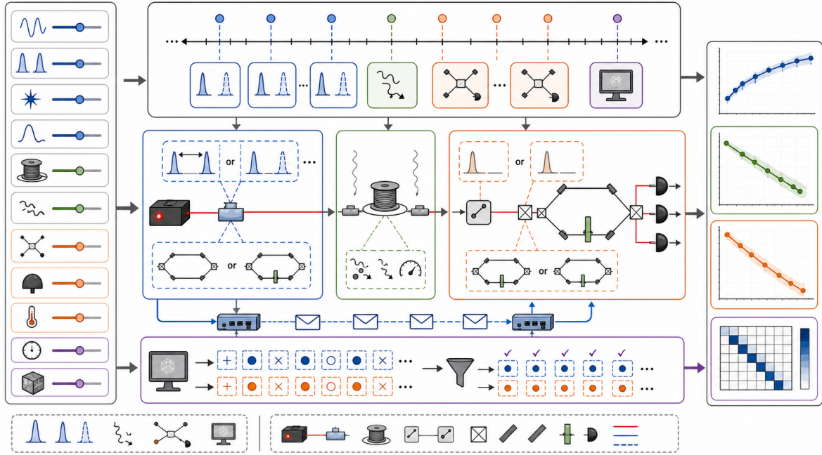
Figura 6.1: Flujo conceptual de simulación de eventos discretos para el enlace BB84 time-bin : parámetros de fuente/canal/receptor, eventos ópticos y clásicos, detección y extracción de métricas. Imagen generada con imagen para esta memoria.
